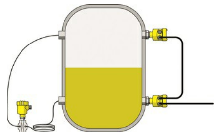
Klassische (links) und elektronische Differenzdruckmessung (rechts).
