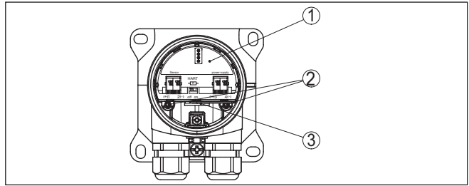
Fig. 2: Zafar los tornillos de sujeción
