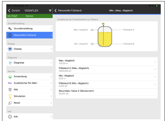
Fig. 20: Voorbeeld van een app-aanzicht - inbedrijfname sensorinregeling
