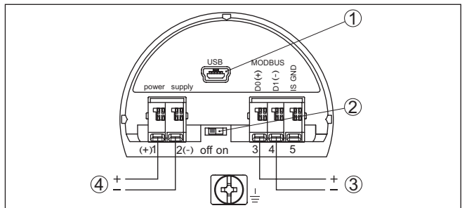
Fig. 12: Aansluitruimte
