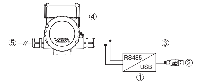
Fig. 23: Aansluiting van de PC via interface-adaptor op de RS 485-kabel
