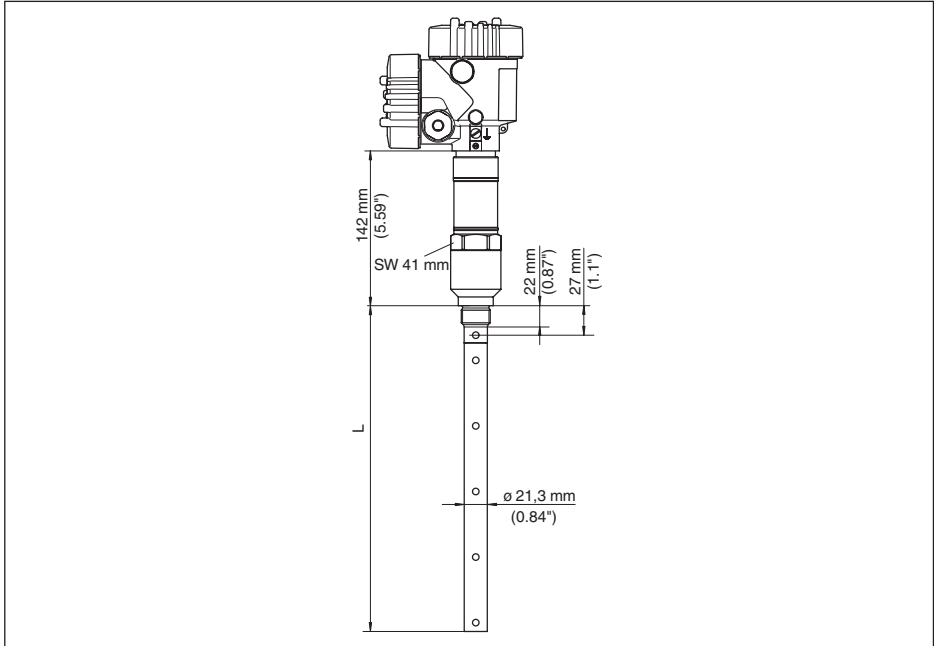
Fig. 36: VEGAFLEX 86, coaxuitvoering met schroefdraad (-20 ... +250 °C/-4 ... +482 °F)
