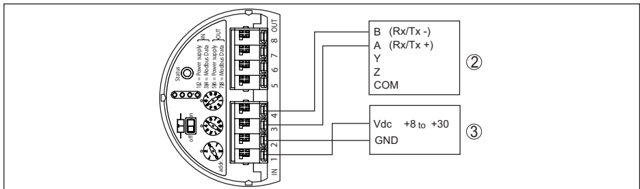
Fig. 34: Aansluiting van de VEGAFLEX 86 op RTU Fisher ROC 809
