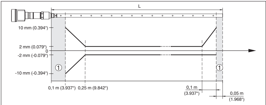
Fig. 31: Meetafwijking VEGAFLEX 86 in coaxuitvoering in product olie (meetlengte tot 1,5 m/4.92 ft)
