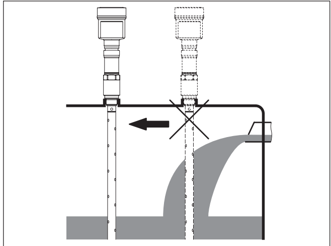
Fig. 6: Montage van de sensor bij instromend product
