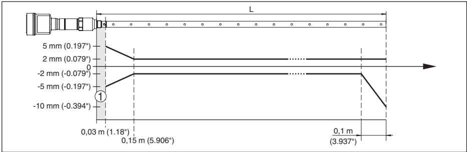
Fig. 29: Meetafwijking VEGAFLEX 86 in coaxuitvoering in product water (meetlengte tot 1,5 m/4.92 ft)
