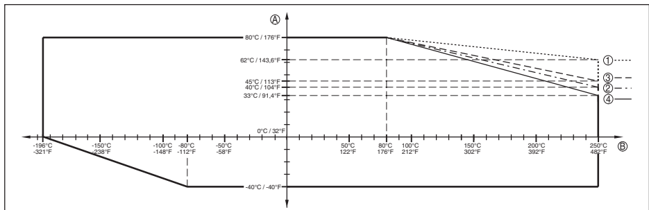
Fig. 33: Omgevingstemperatuur - procestemperatuur standaarduitvoering
