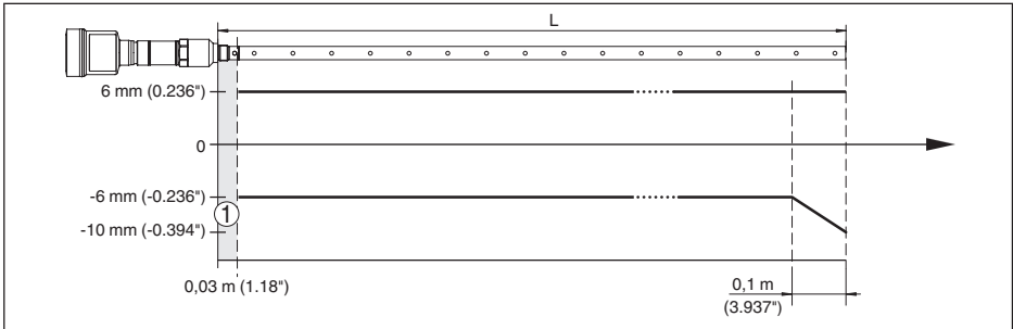
Fig. 30: Meetafwijking VEGAFLEX 86 in coaxuitvoering in product water (meetlengte tot 6 m/19.69 ft)
