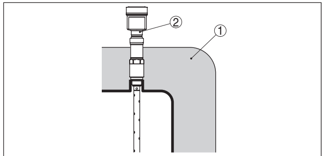
Fig. 8: Montage van het instrument in geïsoleerde tanks.
