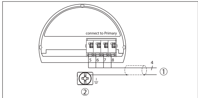
Figura 3: Schema di collegamento VEGABAR 87 secondary device
