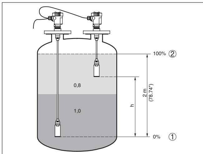
Figura 7: Esempio di parametrizzazione taratura di min./max. per misura d'interfaccia
