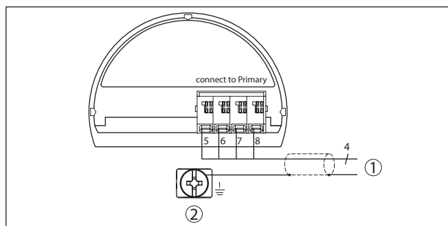
Figura 3: Schema di collegamento VEGABAR 86 secondary device
