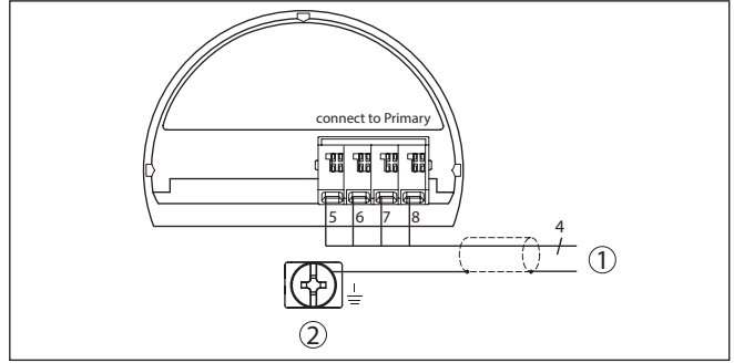
Res. 3: Bağlantı planı VEGABAR 86 arabirim cihazı
