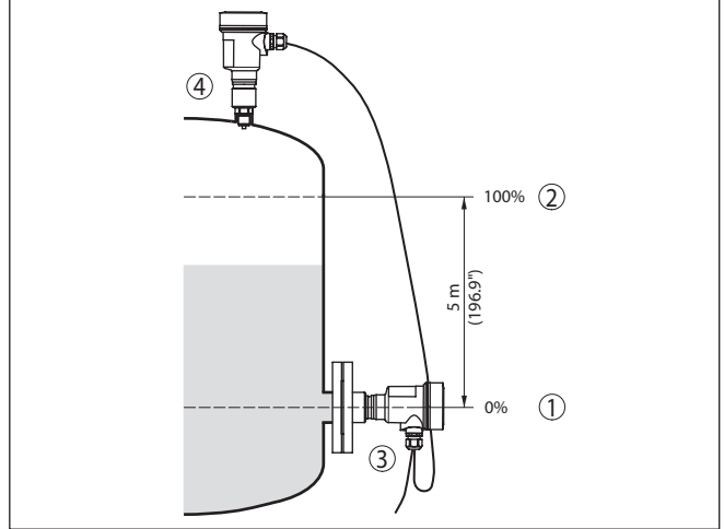
Res. 5: Parametrelere örneği Min. seviyeleme / Maks. seviyeleme Seviye ölçümü
