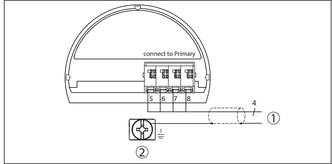
Res. 3: Bağlantı planı VEGABAR 83 arabirim cihazı
