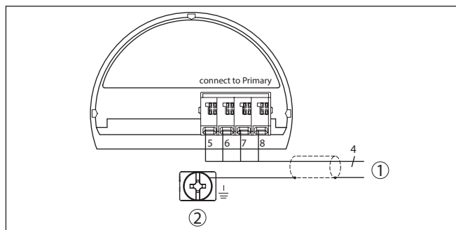
Rys. 3: Schemat przyłączy VEGABAR 82 sondy Secondary
