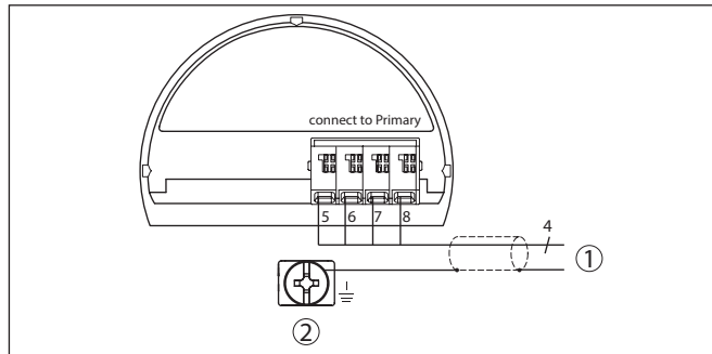
Rys. 3: Schemat przyłączy VEGABAR 81 sondy Secondary
