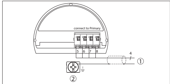
Fig. 3: Plan de raccordement VEGABAR 81 appareil secondaire
