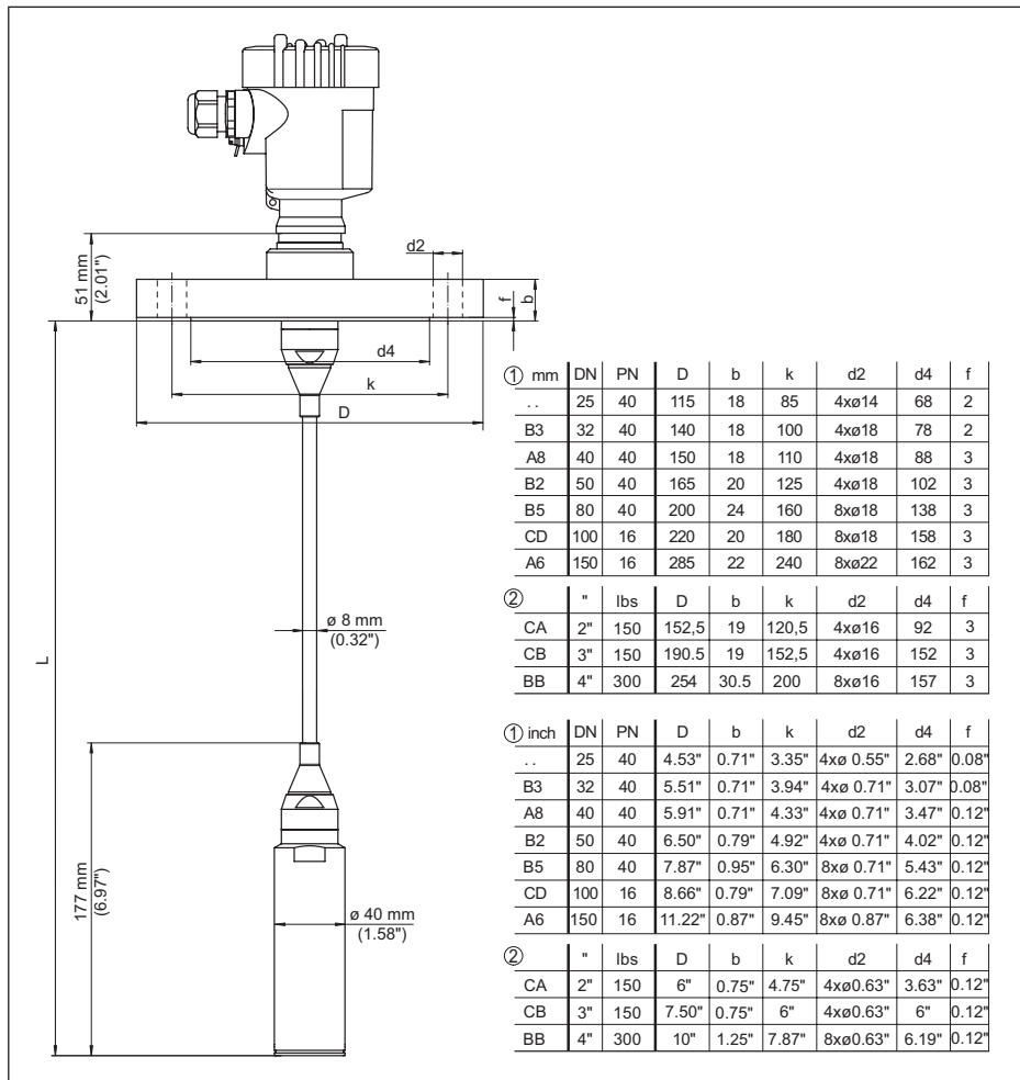
Fig. 30: VEGABAR 87, conexão com flange
