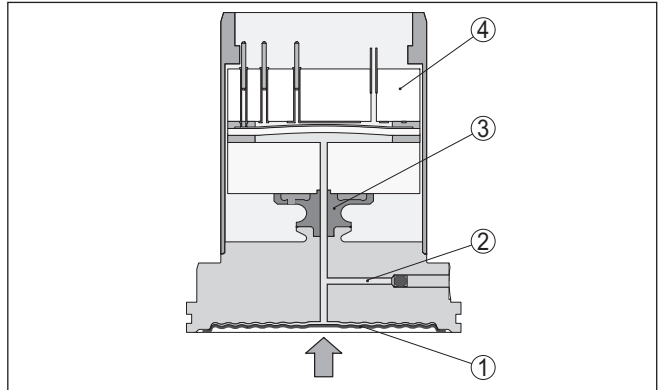
Fig. 2: Estrutura da célula de medição METECC® no VEGABAR 87
