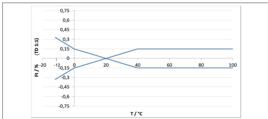
Fig. 24: Erro de temperatura básico F_{TBasis} com TD 1 : 1
