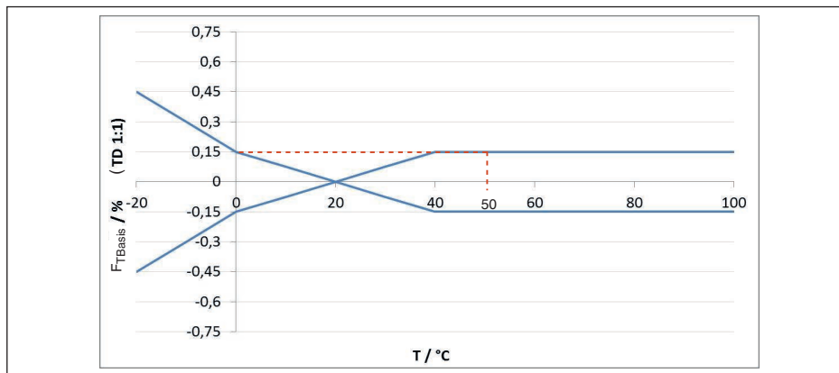
Fig. 25: Cálculo do erro de temperatura básica para o exemplo acima F_{TBasis} = 0,15\% :
