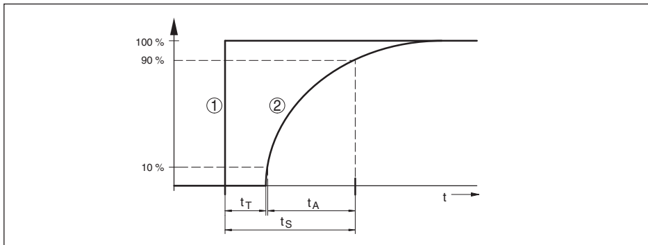
Fig. 23: Comportamento em caso de alteração repentina da grandeza do processo. t_T : tempo morto; t_A : tempo de elevação; t_S : tempo de resposta do salto
