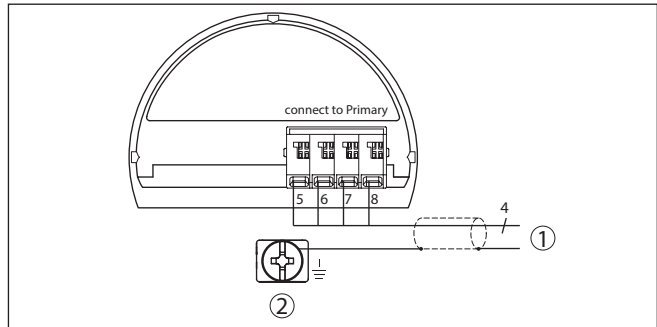
Fig. 15: Esquema de ligações VEGABAR 87 Dispositivo secundário
