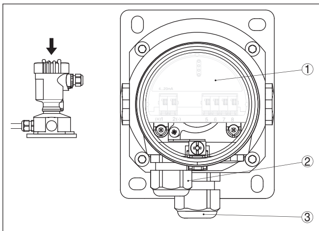
Fig. 17: Compartimento do sistema eletrônico e de conexão
