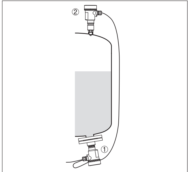
Fig. 2: Ejemplo presión diferencial electrónica para la medición de nivel en depósitos presurizados
