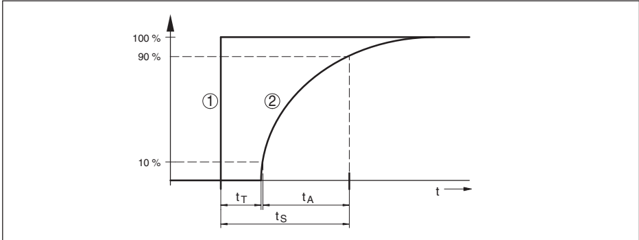
Fig. 23: Comportamiento con variación brusca de las variables de proceso. t_T : tiempo muerto; t_A : tiempo de subida; t_S : tiempo de respuesta gradual
