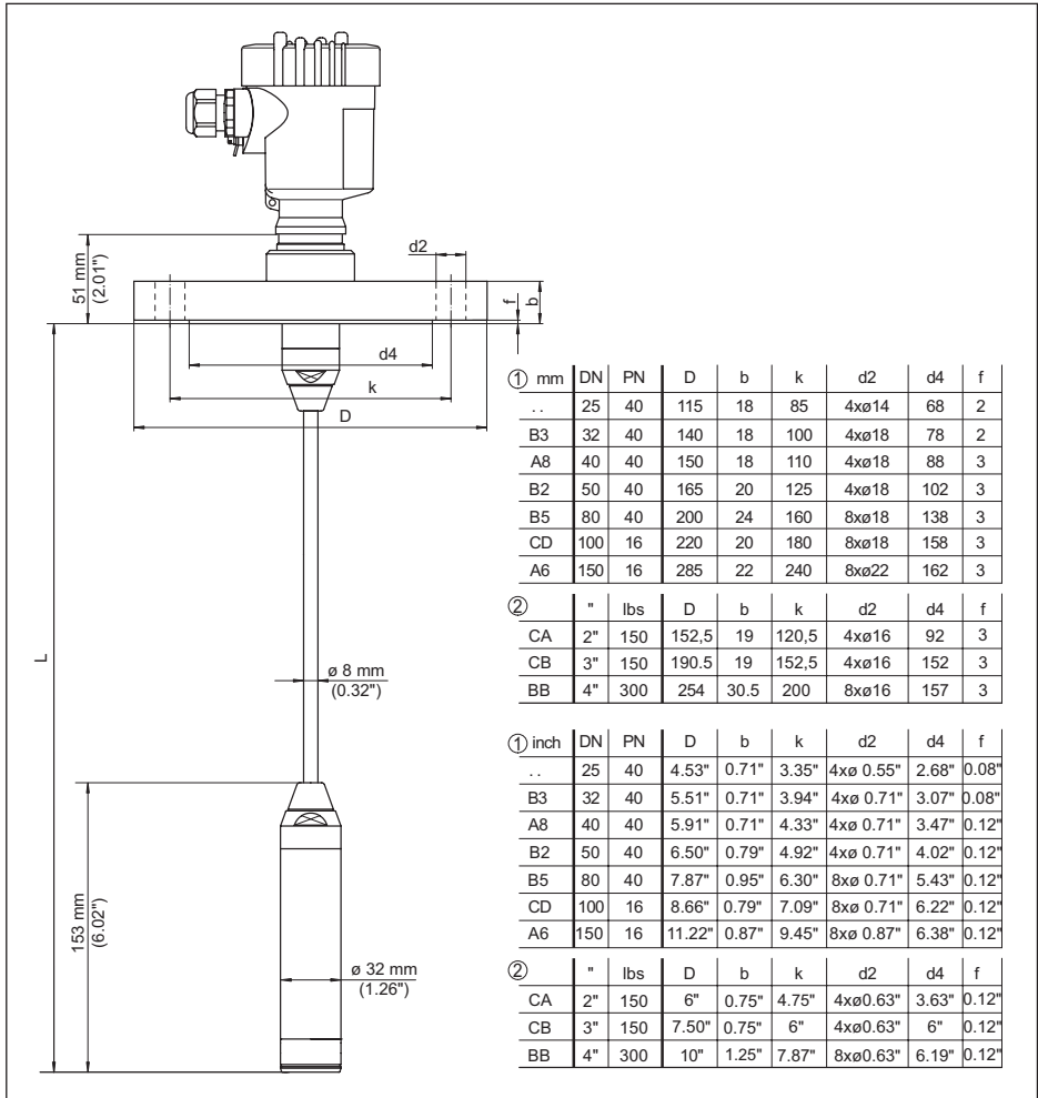
Fig. 32: VEGABAR 86, conexión de brida (ejemplo: transductor de medición de 32 mm)
