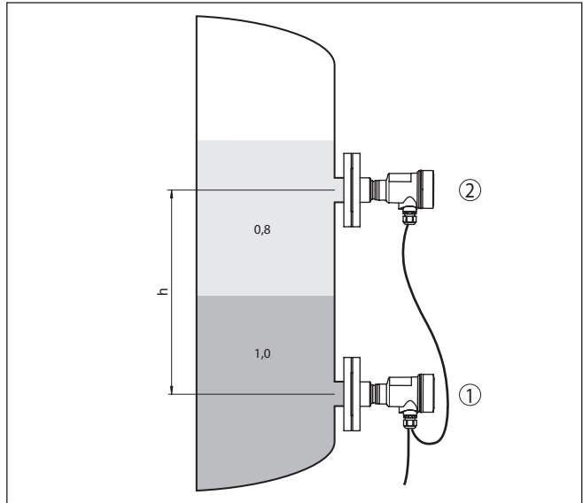
Fig. 11: Configuración de medición para medición de interfase, h = Distancia entre ambos puntos de medición
