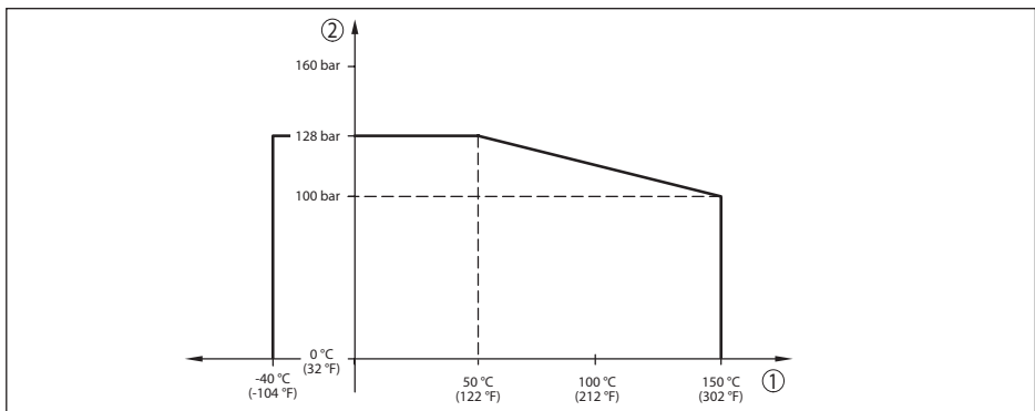
Fig. 25: Reducción de temperatura VEGABAR 81, conexiones a proceso aleación 400 (2.4360)
