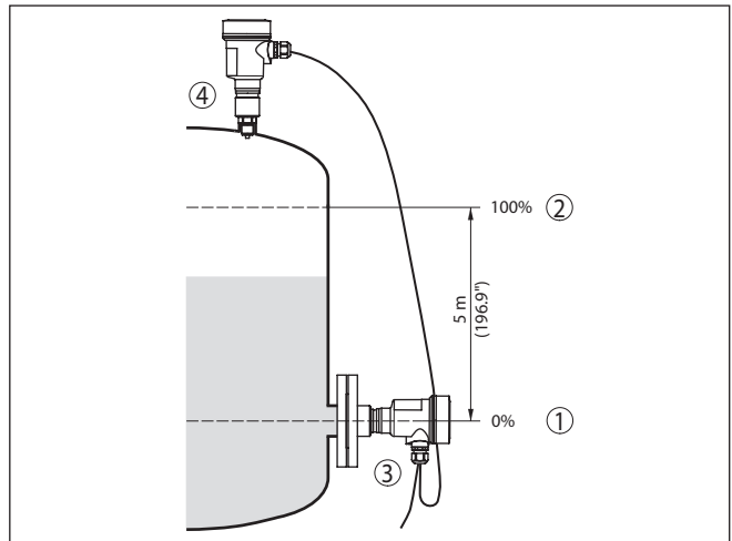
Fig. 22: Ejemplo de parametrización ajuste mín./máx. medición de nivel
