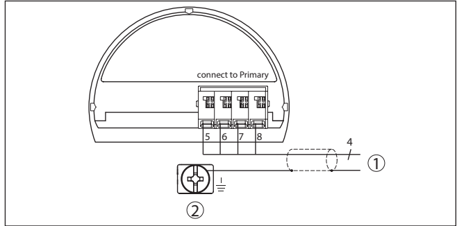
Fig. 16: Esquema de conexiones VEGABAR 81 dispositivo secundario
