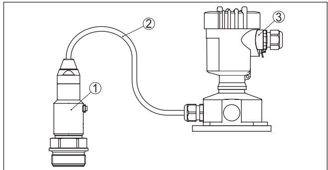
Fig. 17: VEGABAR 81 en versión IP68 25 bar con salida de cable axial, carcasa externa
