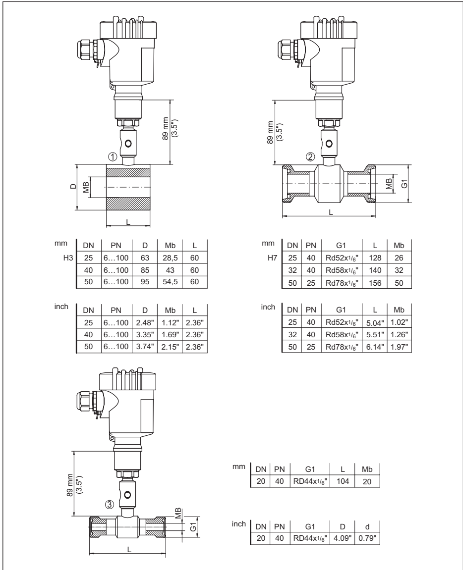
Fig. 29: VEGABAR 81 - Separador tubular
