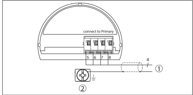
Fig. 20: Esquema de conexiones VEGABAR 81 dispositivo secundario
