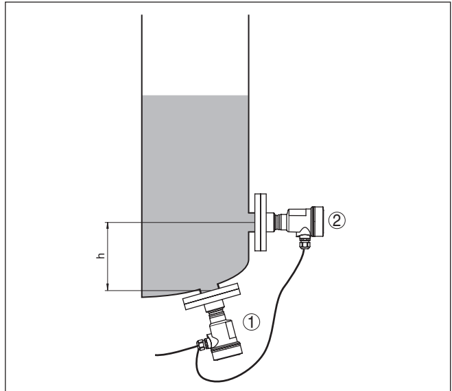
Fig. 13: Configuración de medición para medición de nivel con compensación de densidad, h = distancia entre ambos puntos de medición
