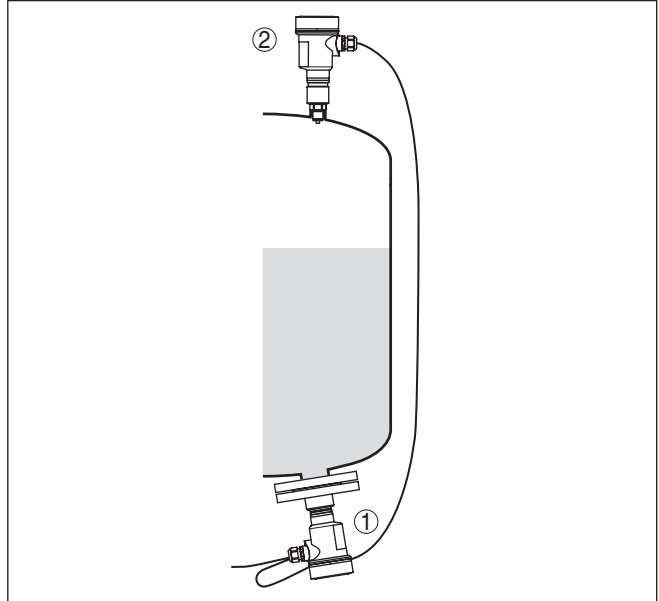
Fig. 9: Configuración de medición para medición de nivel en depósito presurizado
