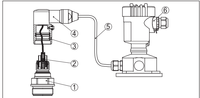
Fig. 23: VEGABAR 81 en versión IP68 25 bar y salida de cable lateral, carcasa externa
