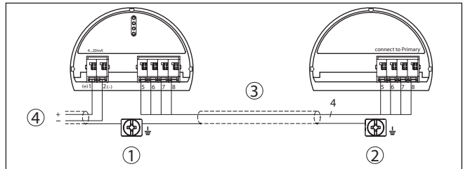
Fig. 21: Ejemplo de conexión presión diferencial electrónica
