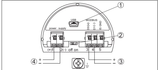
Fig. 6: Compartimiento de conexiones
