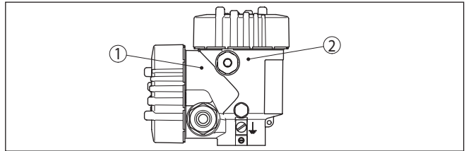
Fig. 4: Posición del compartimiento de conexiones (Electrónica Modbus) y el compartimiento de la electrónica (Electrónica del sensor)
