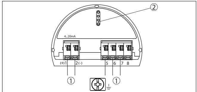
Fig. 5: Elektronicaruimte - tweekamerbehuizing
