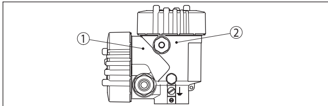
Figura 4: Posizione del vano di connessione (elettronica Modbus) e del vano dell'elettronica (elettronica sensore)
