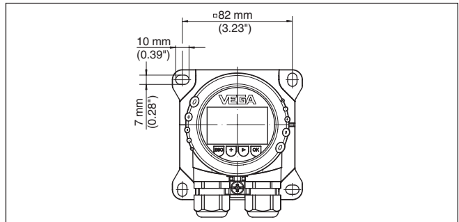
Fig. 3: Dimensions des perçages VEGADIS 82 pour le montage mural
