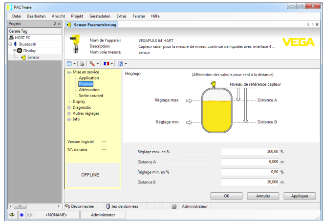
Fig. 19: Exemple de masque DTM
