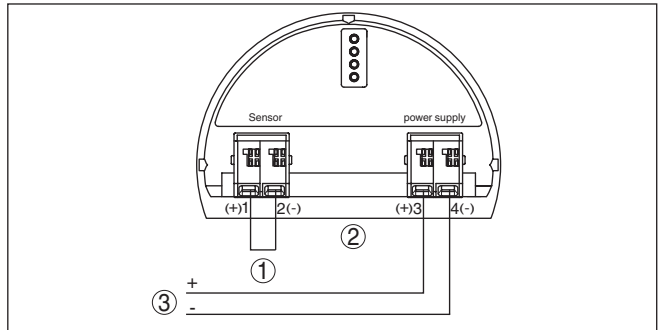
Fig. 12: Pont sur les bornes 1 et 2 sur le VEGADIS 82
