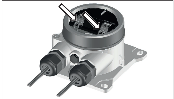
Fig. 8: Étapes de raccordement 5 et 6
