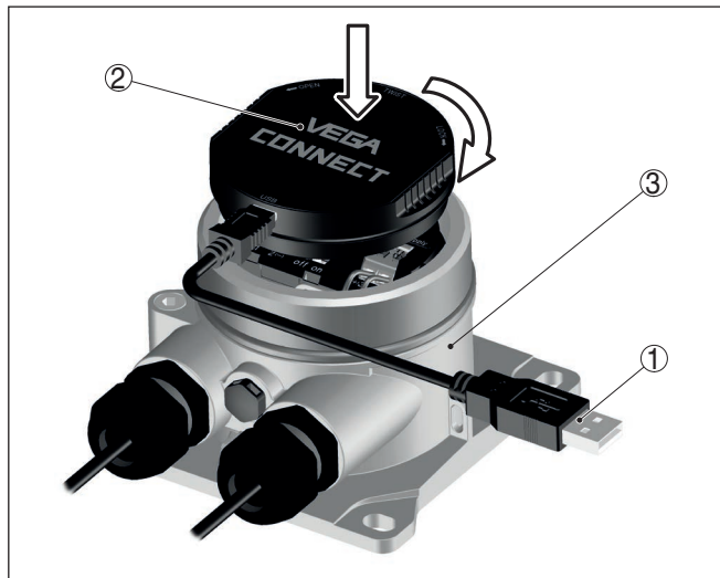
Fig. 18: Raccordement du PC via l'adaptateur d'interfaces
