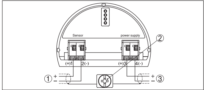
Fig. 9: Schéma de raccordement VEGADIS 82 pour capteurs 4 ... 20 mA
