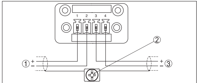
Fig. 10: Schéma de raccordement VEGADIS 82 pour capteurs 4 ... 20 mA - montage encastré
