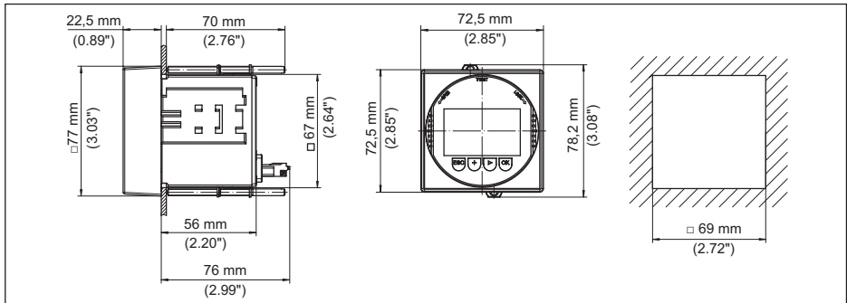
Fig. 21: VEGADIS 82 avec boîtier en plastique pour montage encastré
