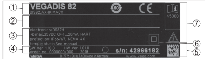
Fig. 1: Présentation de la plaque signalétique (exemple)
