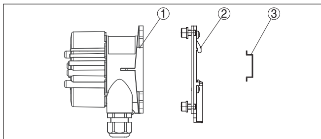
Fig. 5: VEGADIS 82 avec boîtier en aluminium ou acier inox pour le montage sur rail
