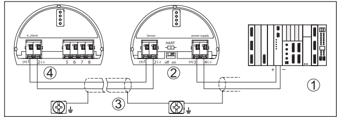
Fig. 15: Exemple de raccordement capteur 4...20 mA et système d'exploitation/API
