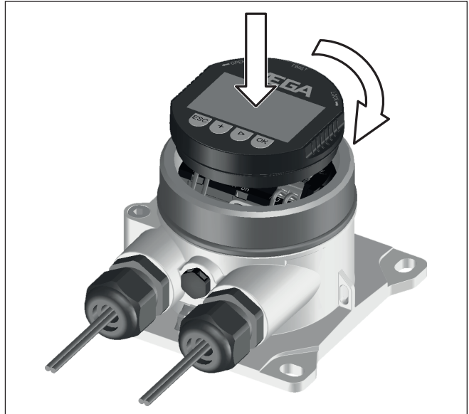
Fig. 16: Montage du module de réglage et d'affichage
