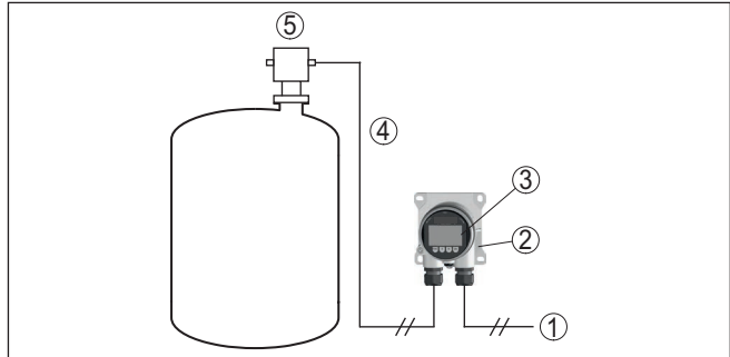
Fig. 2: Raccordement du VEGADIS 82 au capteur
