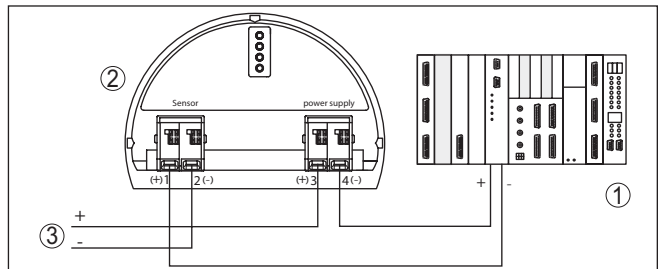
Fig. 14: Raccordement du VEGADIS 82 comme affichage externe à un capteur quatre fils avec sortie 4...20 mA active et système d'exploitation/API supplémentaire
