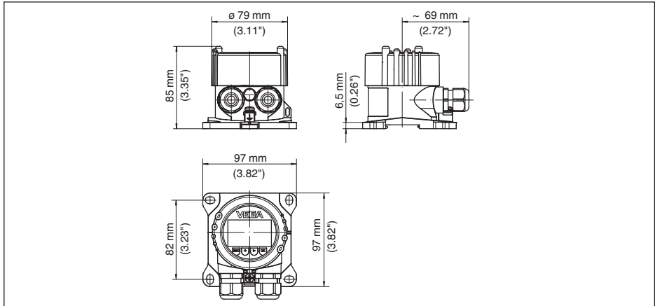
Fig. 20: VEGADIS 82 avec boîtier en plastique
