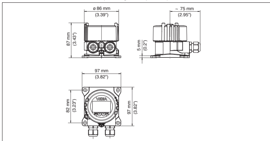
Fig. 23: VEGADIS 82 avec boîtier en acier inox (moulage cire-perdue)
