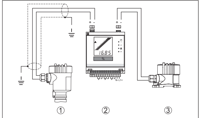
Fig. 11: Raccordement du VEGADIS 82 à l'unité de commande comme affichage externe
