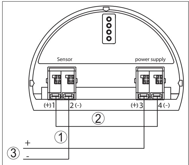
Fig. 13: Raccordement du VEGADIS 82 comme affichage externe à un capteur quatre fils avec sortie 4...20 mA active
