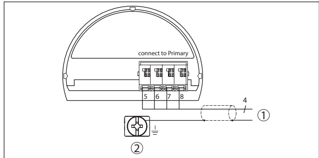
Fig. 3: Esquema de conexiones VEGABAR 87 dispositivo secundario
