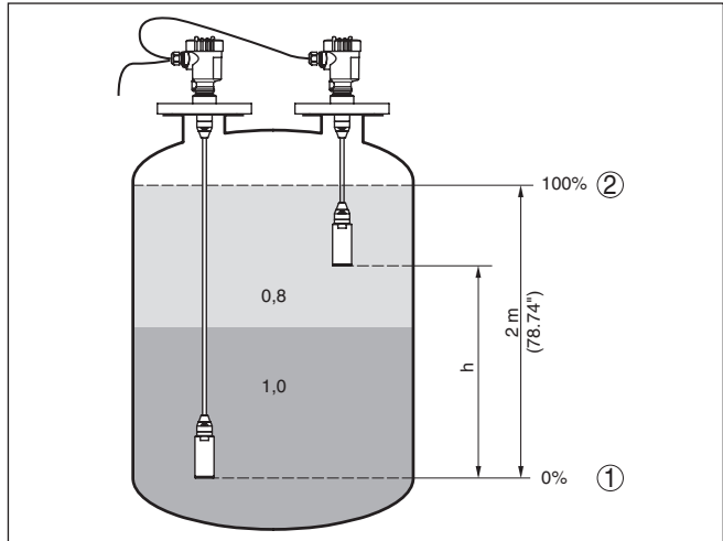
Fig. 5: Parametrevoorbeeld min./max.-inregeling scheidingslaagmeting
