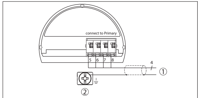
Figura 3: Schema di collegamento VEGABAR 87 secondary device
