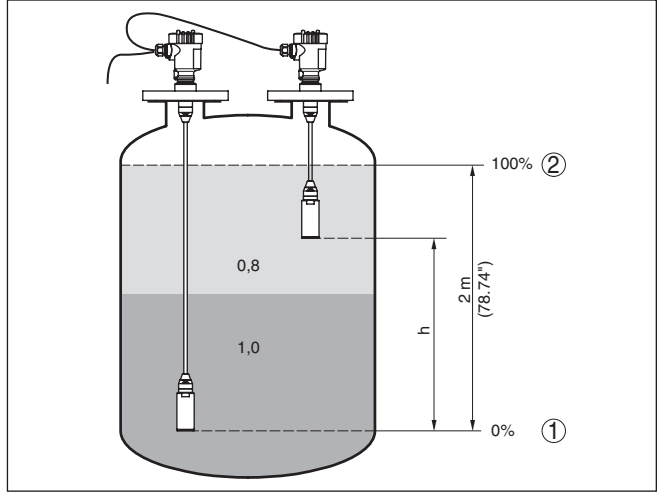
Res. 5: Parametreleme örneği Min. seviyeleme / Maks. seviyeleme Ayırma katmanı ölçümü
