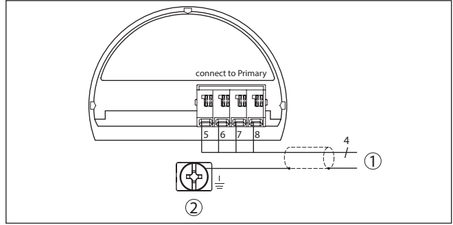
Res. 3: Bağlantı planı VEGABAR 86 arabirim cihazı
