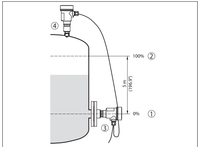
Fig. 5: Parametreevoorbeeld min.-/max.-inregeling niveaumeting
