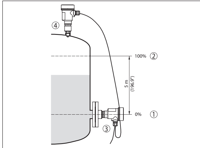
Rys. 5: Przykład parametrów do kompensacji min./max. pomiaru poziomu napełnienia
