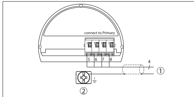
Fig. 3: Esquema de conexiones VEGABAR 81 dispositivo secundario
