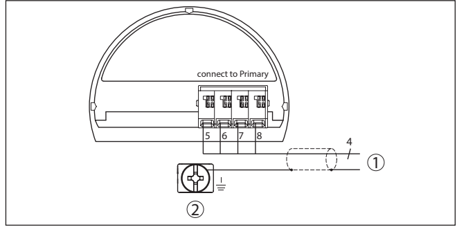
Res. 3: Bağlantı planı VEGABAR 81 arabirim cihazı
