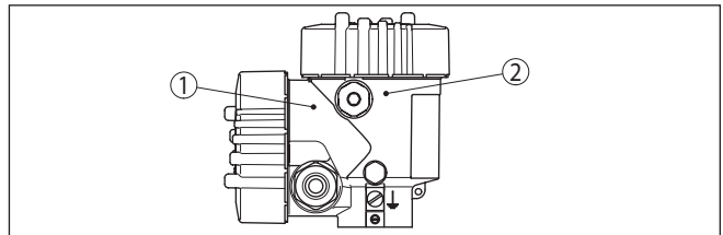
Fig. 3: Position du compartiment de raccordement (électronique du Modbus) et du compartiment de l'électronique (électronique du capteur)
