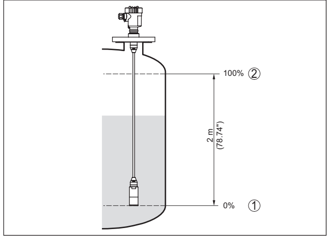
Res. 6: Parametreleme örneği Min. seviyeleme / Maks. seviyeleme Seviye ölçümü
