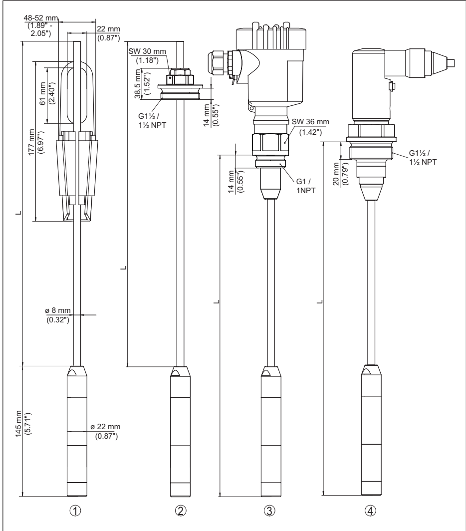
Res. 32: VEGABAR 86, ölçüm sondası (22 mm)
