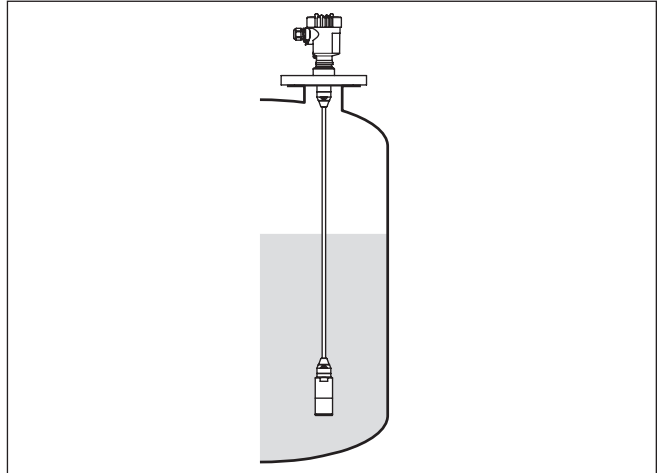
Res. 2: VEGABAR 86'li dolmuş seviyesi ölçümü
