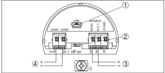
Res. 14: Bağlantı bölgesi
