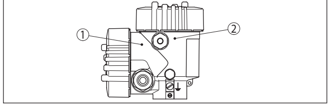
Res. 9: Bağlantı mekanının konumu (Modbus elektroniği) ve elektronik mekan (sensör elektroniği)
