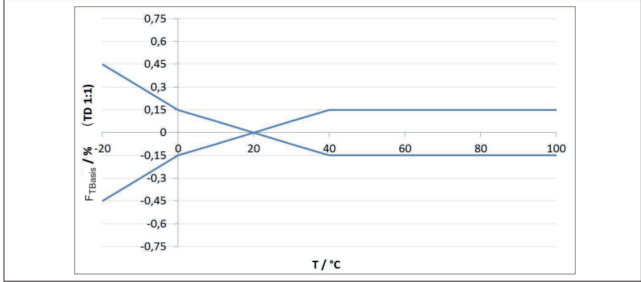
Res. 26: Temel sıcaklık hatası TD 1 : 1'de F_{TBasic}
