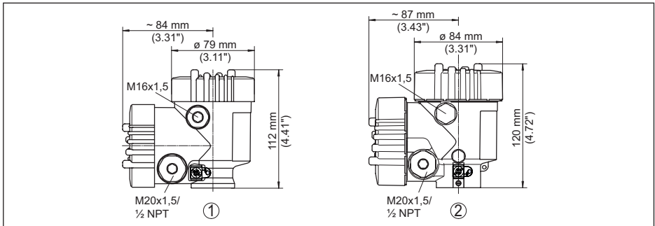
Res. 29: Gövdenin ebatları (entegre gösterge ve kontrol modüllü gövde yüksekliği 9 mm/0.35 in ya da 18 mm/0.71 in değeri kadar artar)
