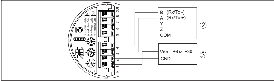
Res. 27: VEGABAR 86'un an RTU Fisher ROC 809'a bağlanması
