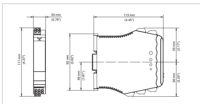
Encombrement VEGATOR 122
