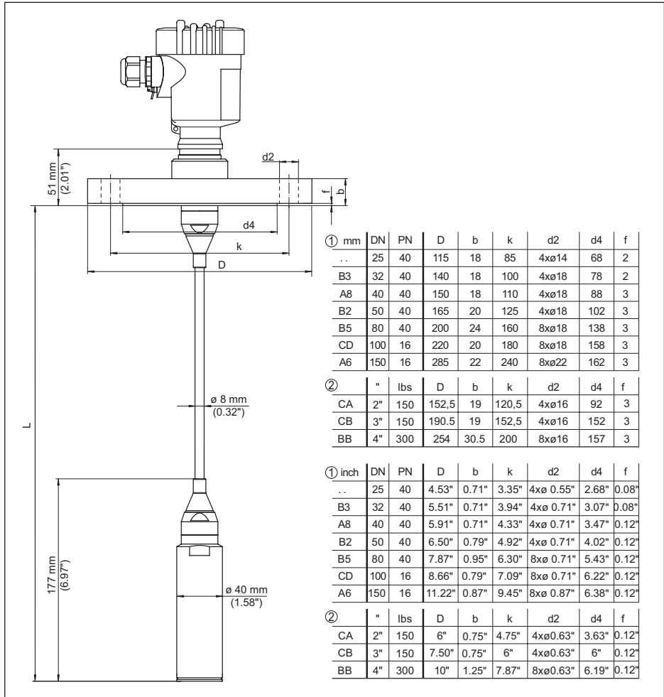
Figura 31: VEGABAR 87, attacco a flangia
