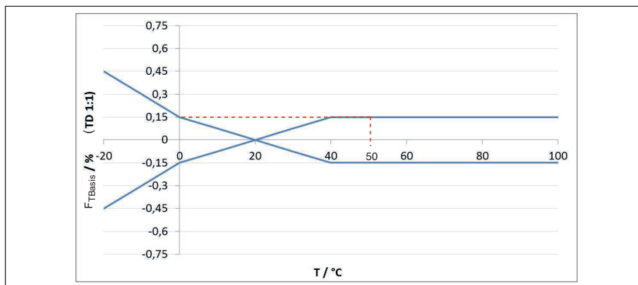
Figura 27: Calcolo dell'errore di temperatura base per il suddetto esempio: F_{TBasis} = 0,15\%
