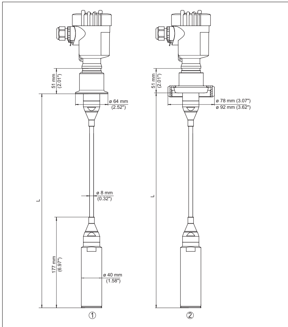
Figura 32: VEGABAR 87, attacchi igienici
