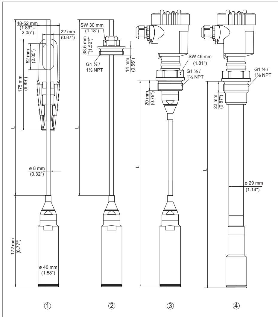
Figura 30: VEGABAR 87 - Attacchi standard
