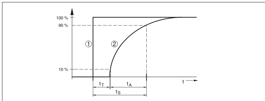
Fig. 23: Comportamento em caso de alteração repentina da grandeza do processo. t_T : tempo morto; t_A : tempo de subida; t_S : tempo de resposta do salto
