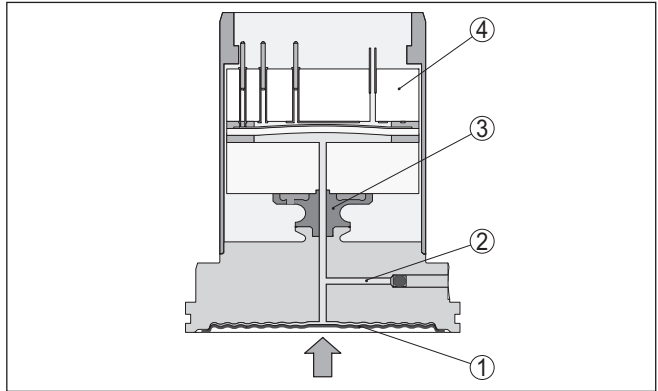
Fig. 2: Estrutura da célula de medição METEC® no VEGABAR 87
