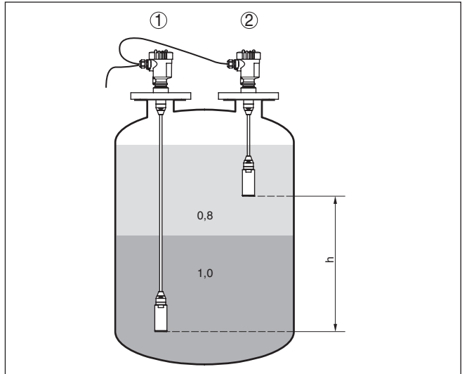
Fig. 9: Configuración de medición para medición de interfase, h = Distancia entre ambos puntos de medición
