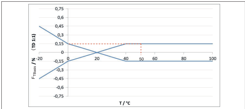
Fig. 24: Determinación del error de temperatura básico para el ejemplo anterior: F_{TBasis} = 0,15 \%
