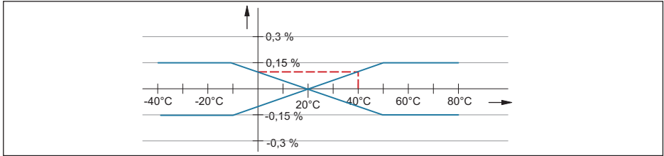
Fig. 25: F_a por variación térmica en la salida de corriente, en este ejemplo= \mathbf{0,1 \%}
