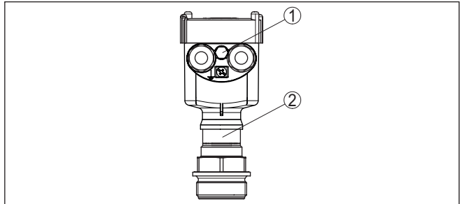
Fig. 6: Posición del elemento de filtrado - Versión hermética al gas
