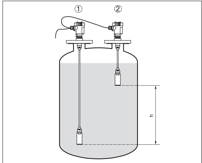
Fig. 10: Configuración de medición para medición de densidad, h = Distancia entre ambos puntos de medición
