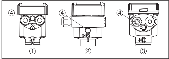
Fig. 5: Posición del elemento de filtrado - versiones No-Ex y Ex ia
