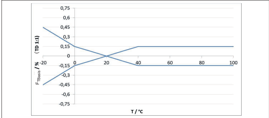
Fig. 23: Error de temperatura básico F_{TBasic} con TD 1 : 1
