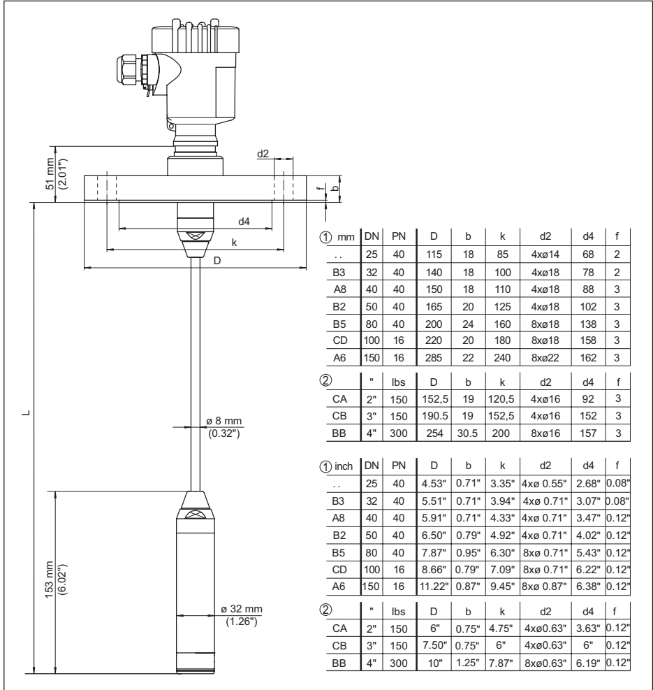
Fig. 31: VEGABAR 86, conexión de brida (ejemplo: transductor de medición de 32 mm)
