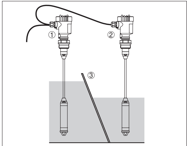
Fig. 8: Configuración de medición para la medición de diferencia de nivel
