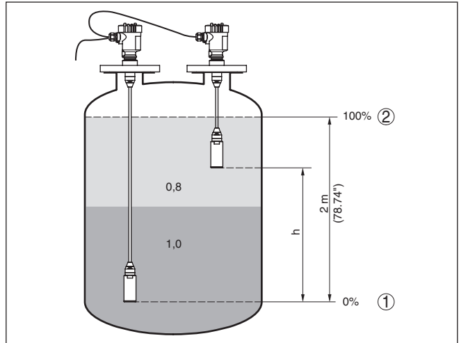
Fig. 20: Ejemplo de parametrización ajuste mín./máx. medición de interfase
