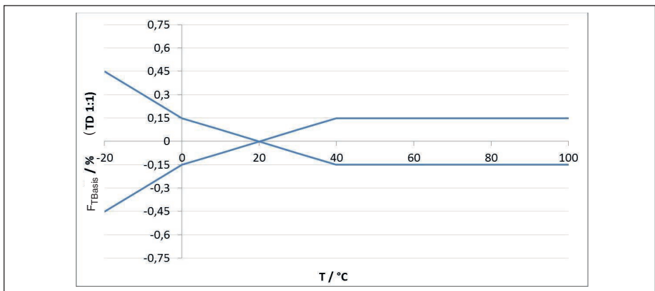
Fig. 23: Basistemperatuurfout F_{TBasis} bij TD 1 : 1
