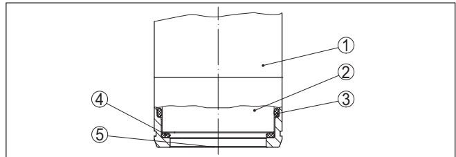
Fig. 2: Vlakke inbouw van de keramische meetcel met dubbele afdichting
