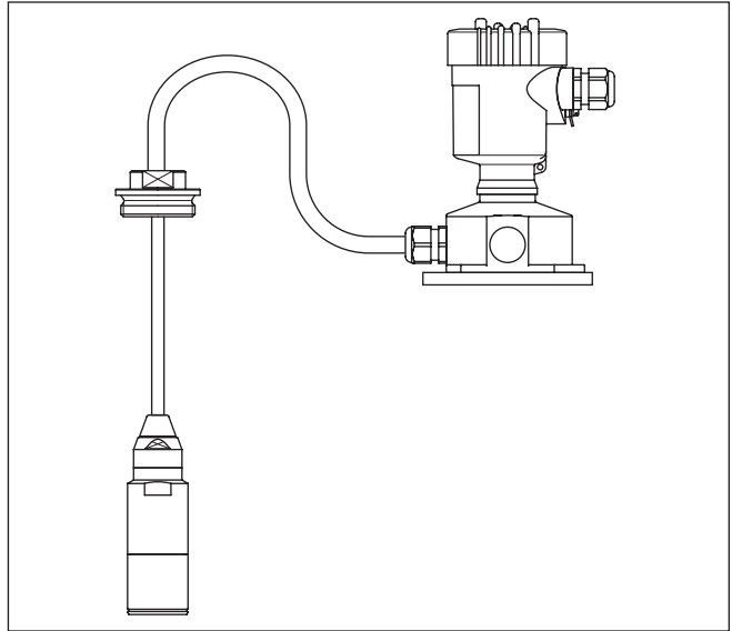
Fig. 15: VEGABAR 86 in IP68-uitvoering 25 bar, niet-Ex en axiale kabeluitgang, externe behuizing
