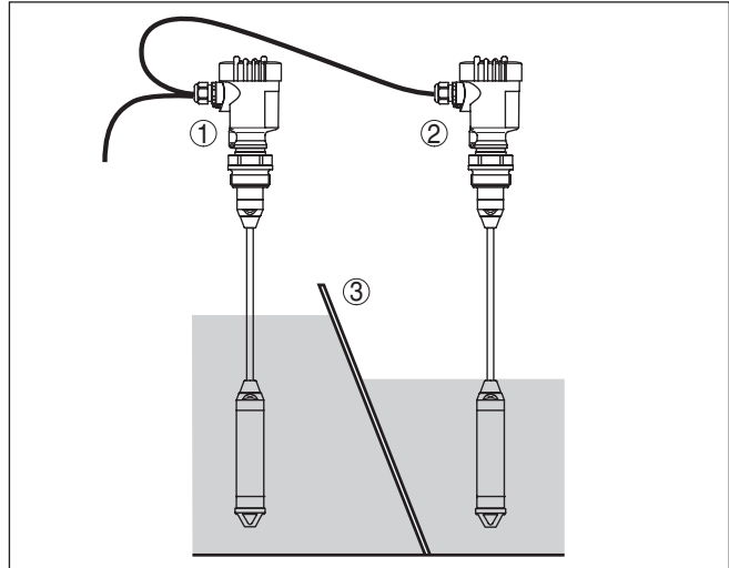
Fig. 8: Meetopstelling bij de niveauverschilmeting
