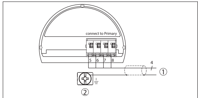
Fig. 14: Aansluitschema VEGABAR 86 secondary device
