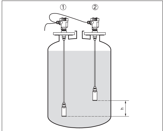
Fig. 11: Meetopstelling bij dichtheidsgecompenseerde niveaumeting, h = afstand tussen de beide meetpunten.
