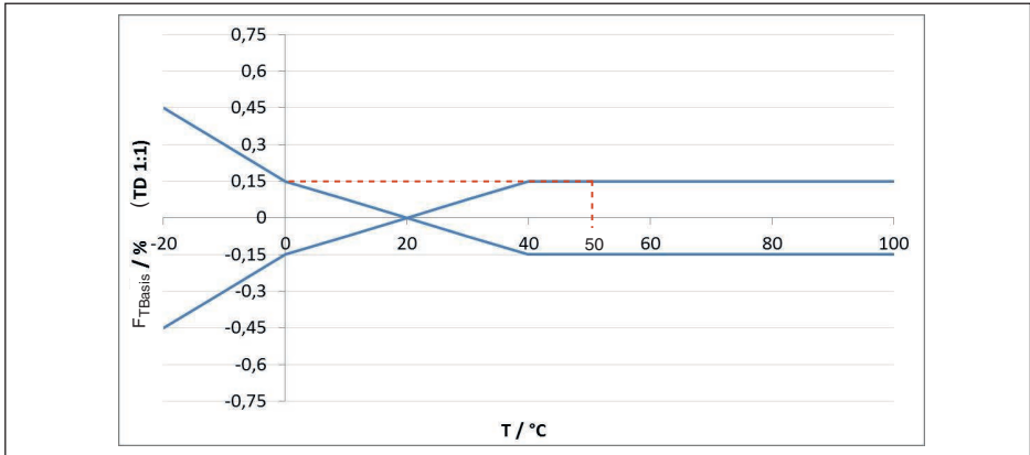
Fig. 24: Bepaling van de basistemperatuurfout voor het voorbeeld boven: F_{TBasis} = 0,15\%
