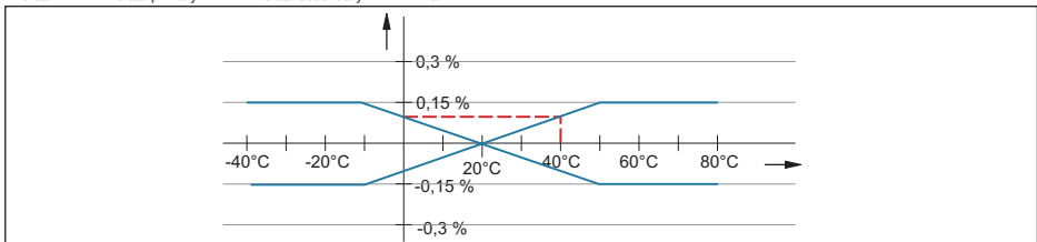
Fig. 25: F_a door thermische verandering van de stroomuitgang, in dit voorbeeld = 0,1 %
