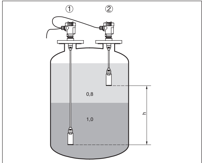
Fig. 9: Meetopstelling bij scheidingslaagmeting, h = afstand tussen de beide meetpunten
