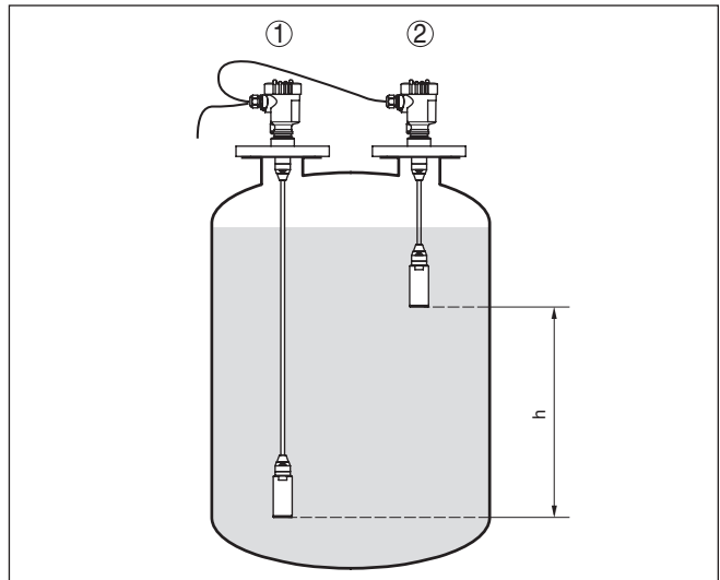
Fig. 10: Meetopstelling bij dichtheidsmeting, h = afstand tussen de beide meetpunten
