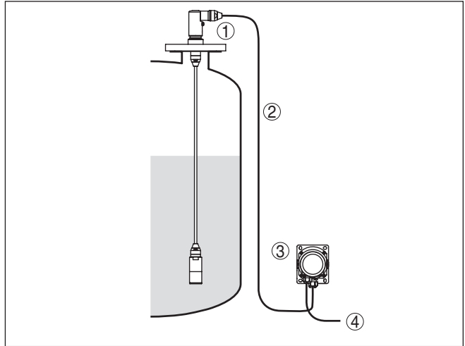
Fig. 12: Opstelling meetplaats, externe behuizing
