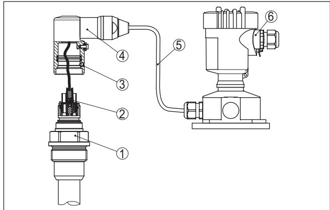
Fig. 21: VEGABAR 86 in IP 68-uitvoering 25 bar en kabeluitgang aan de zijkant, externe behuizing
