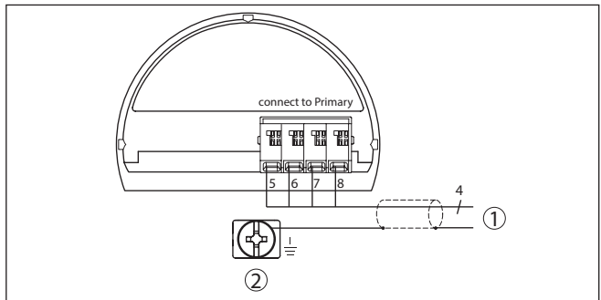
Fig. 18: Aansluitschema VEGABAR 86 secondary device
