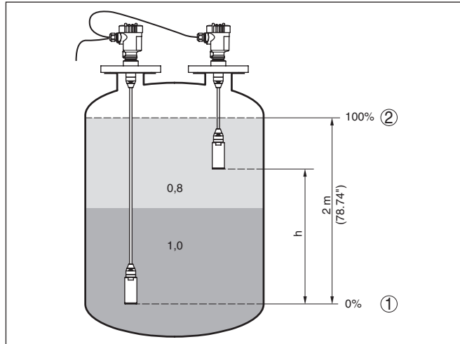
Fig. 20: Parametrevoorbeeld min./max.-inregeling scheidingslaagmeting
