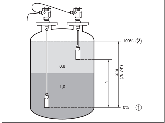
Res. 20: Parametreleme örneği Min. seviyelere / Maks. seviyelere Ayırma katmanı ölçümü
