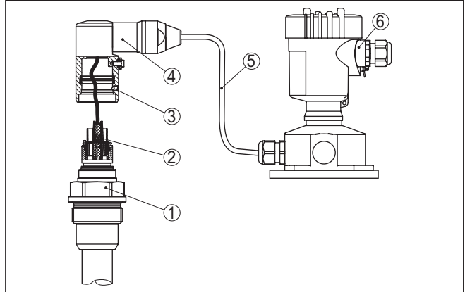
Res. 21: IP 68 modelinde (25 bar) ve yan taraftan kablo çıkışında, dış gövde VEGABAR 86
