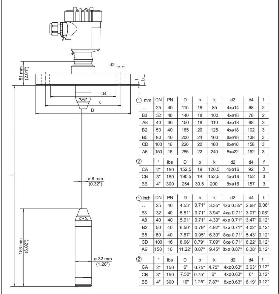
Res. 31: VEGABAR 86, flanş bağlantısı (32 mm'lik ölçüm değeri algılayıcısı örneği)
