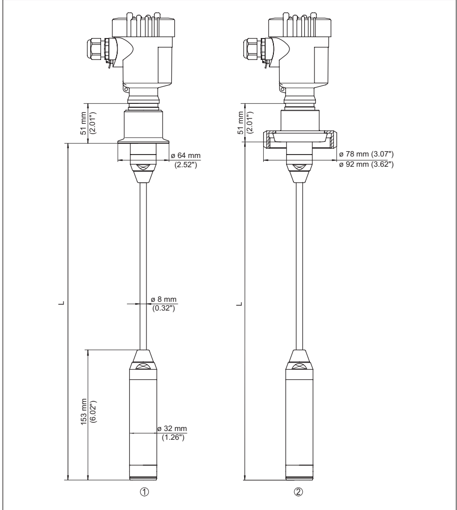
Res. 32: VEGABAR 86, hijyenik bağlantılar
