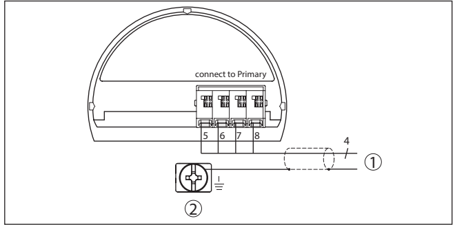
Res. 18: Bağlantı planı VEGABAR 86 arabirim cihazı
