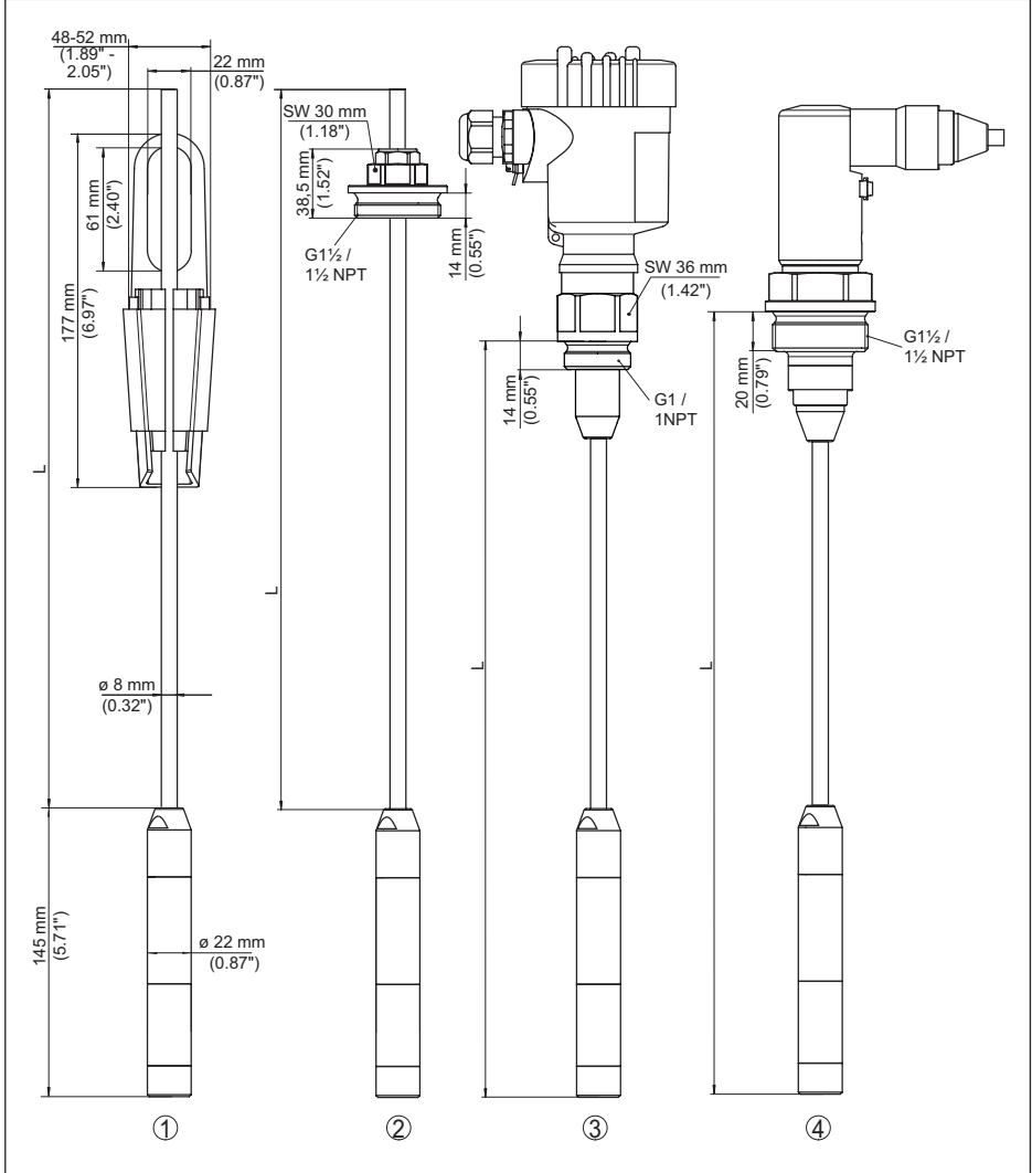
Res. 29: VEGABAR 86, ölçüm sondası (22 mm)
