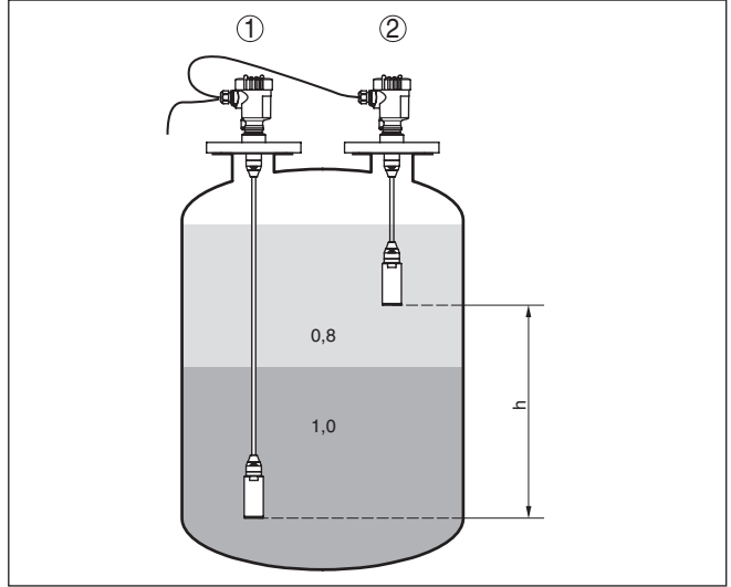
Res. 9: Ayrırma katmanı ölçümü alınacağıında kullanılacak ölçüm yöntemi, h = İki ölçüm noktası arasındaki uzaklık
