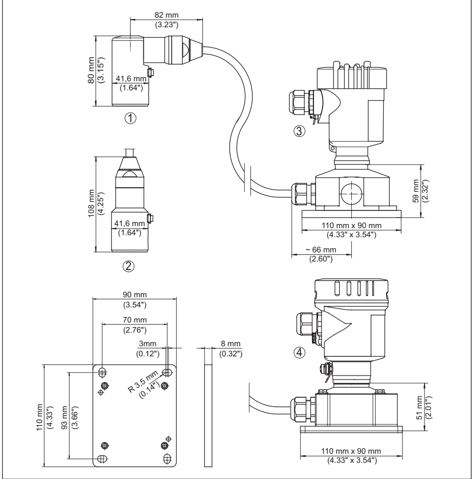
Res. 27: VEGABAR 86, dış gövdeli IP68 modeli
