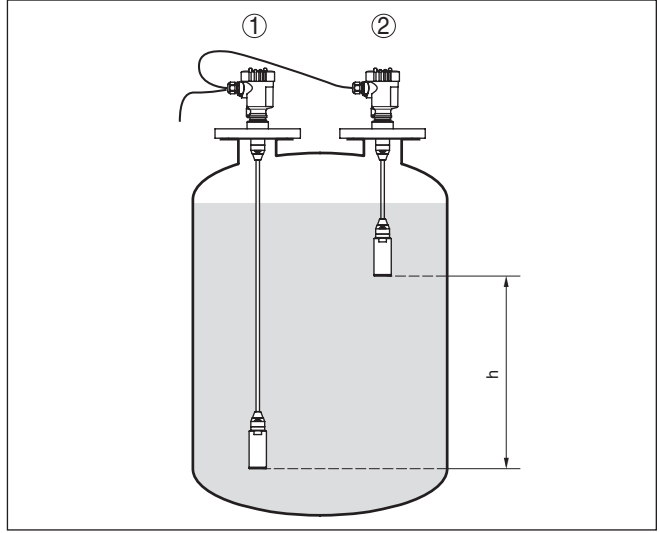
Res. 10: Yoğunluk ölçümü alınacağında kullanılacak ölçüm yöntemi, h = İki ölçüm noktası arasındaki uzaklık
