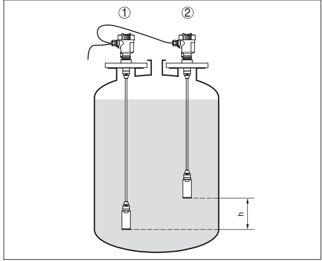
Res. 11: Yoğunluğu dengelenmiş seviye ölçümü düzeni, h = iki ölçüm noktası arasındaki mesafe
