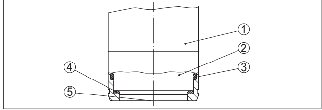
Res. 2: Seramik ölçüm hücresinin ikili contayla yüzey seviyesinde yerleştirilmesi
