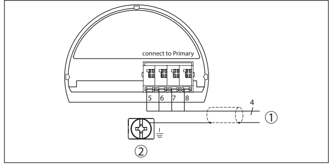
Res. 14: Bağlantı planı VEGABAR 86 ararım cihazı
