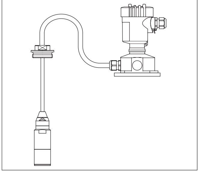
Res. 15: IP68 modelinde (25 bar), Ex olmayan ve eksen yönünde kablo çıkışında, dış gövdeli VEGABAR 86
