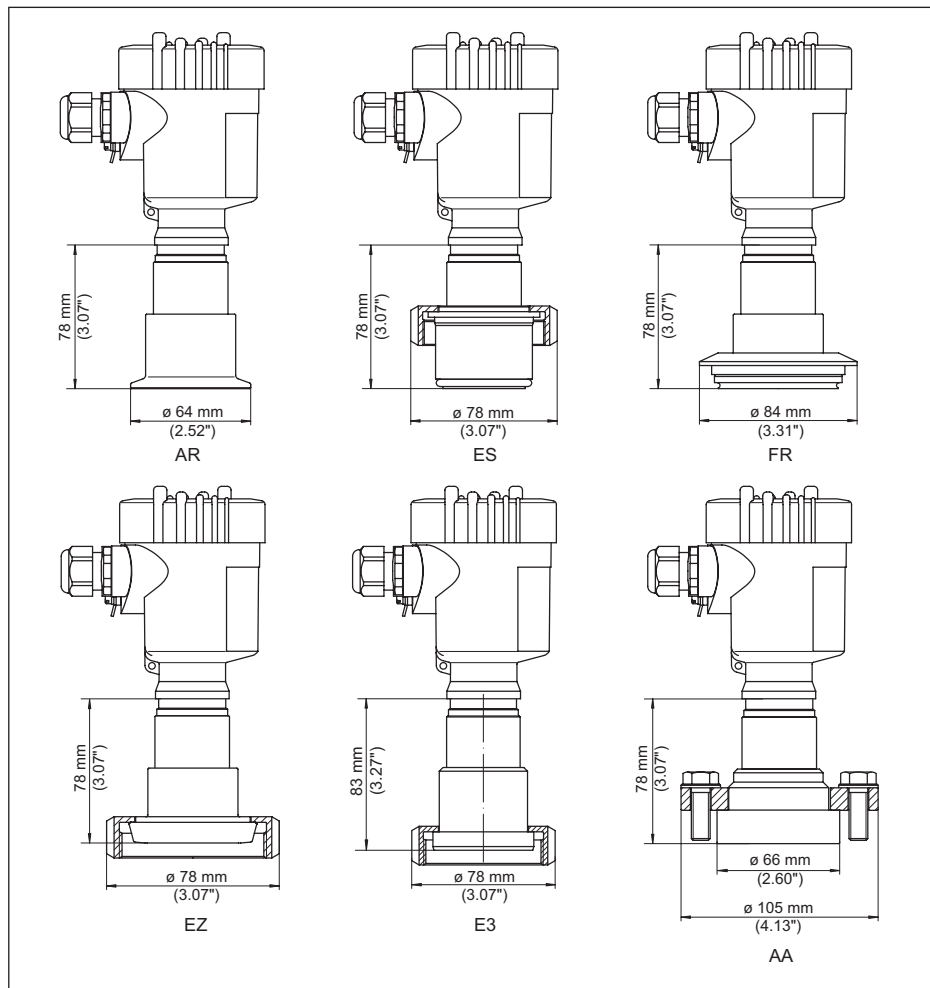
Fig. 38: VEGABAR 83, conexión higiénica +150 °C (celda de medición METEC®)
