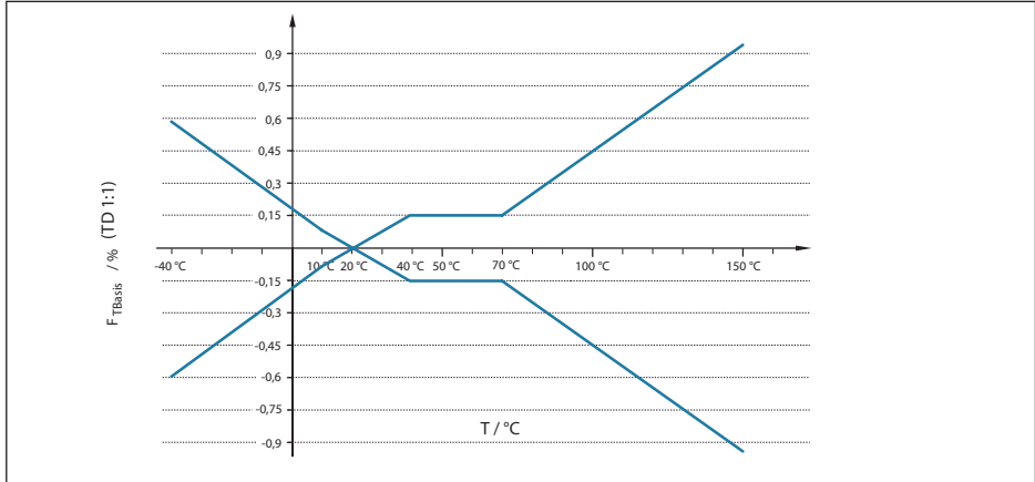
Fig. 23: Error de temperatura básico F_{TBasic} con TD 1 : 1
