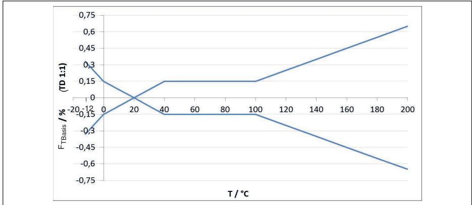
Fig. 24: Error de temperatura básico F_{TBasis} con TD 1 : 1
