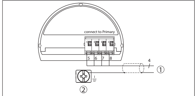
Fig. 14: Esquema de conexiones VEGABAR 83 dispositivo secundario
