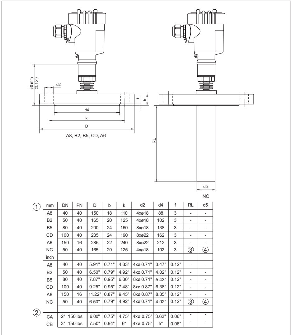
Fig. 39: VEGABAR 83, conexión de brida +150 °C (Celda de medida piezorresistiva/galga extensométrica)
