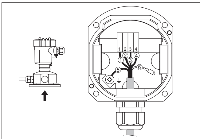
Fig. 17: Conexión del módulo de proceso en el zócalo de la carcasa
