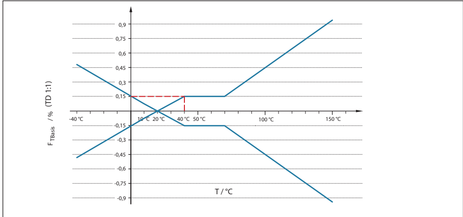
Fig. 30: Determinación del error de temperatura básico para el ejemplo anterior: F_{TBasis} = 0,15\%
