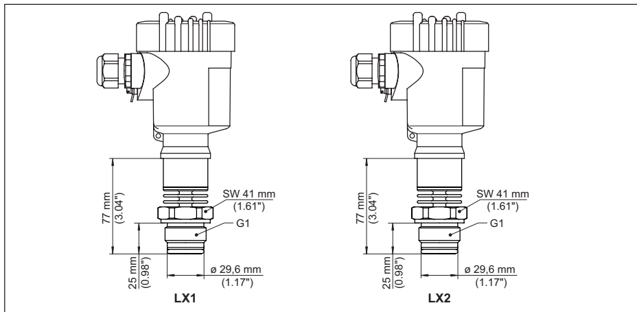
Fig. 36: VEGABAR 83, rosca para adaptador higiénico
