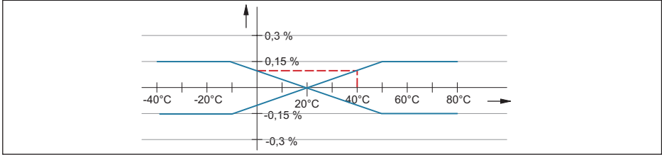
Fig. 31: F_a por variación térmica en la salida de corriente, en este ejemplo = 0,1 %
