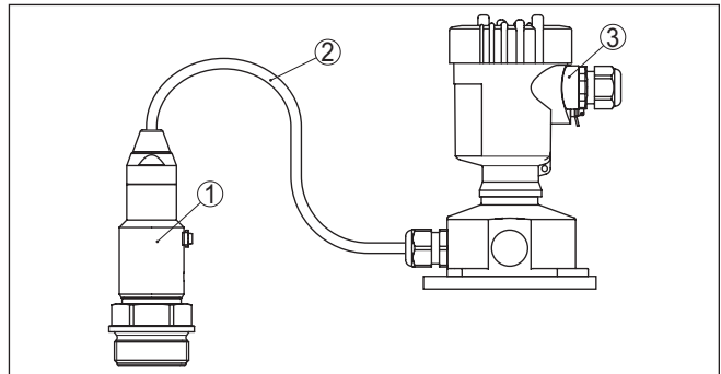
Fig. 15: VEGABAR 83 en versión IP68 25 bar con salida de cable axial, carcasa externa
