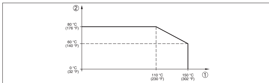
Fig. 27: Reducción de temperatura VEGABAR 83, versión hasta +150 °C (+302 °F)
