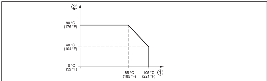
Fig. 25: Reducción de temperatura VEGABAR 83, versión hasta +105 °C (+221 °F)
