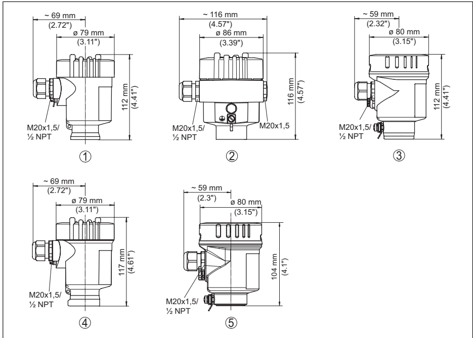
Fig. 32: Variantes de carcasa con tipo de protección IP66/IP67 e IP66/IP68 (0,2 bar), (con el módulo de visualización y configuración montado aumenta la altura de la carcasa en 9 mm/0.35 in o 18 mm/0.71 in)
