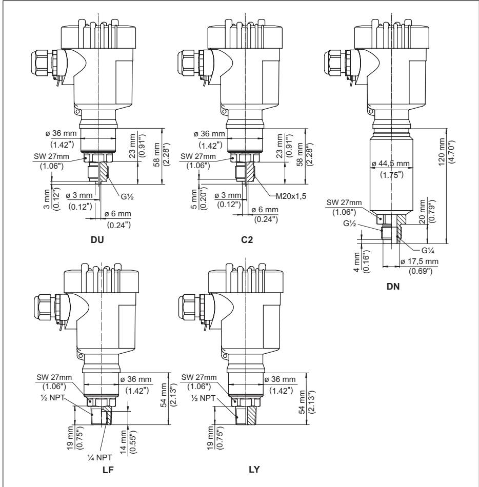
Fig. 34: VEGABAR 83, racor roscado no frontal rasante
