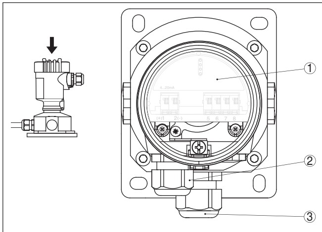
Fig. 16: Compartimento de la electrónica y de conexiones
