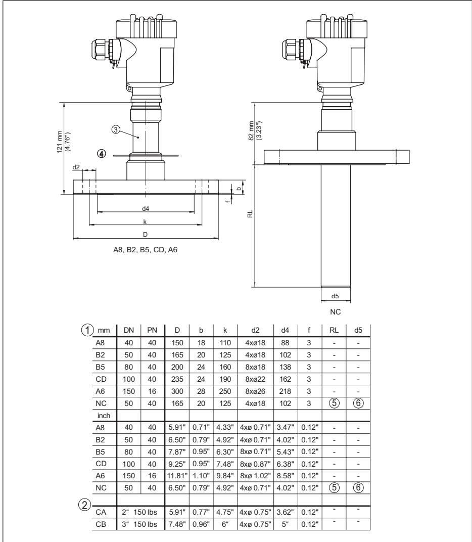
Fig. 40: VEGABAR 83, conexión de brida +180 °C/+200 °C (celda de medida METEC®)
