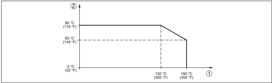
Fig. 28: Reducción de temperatura VEGABAR 83, versión hasta +180 °C (+356 °F)
