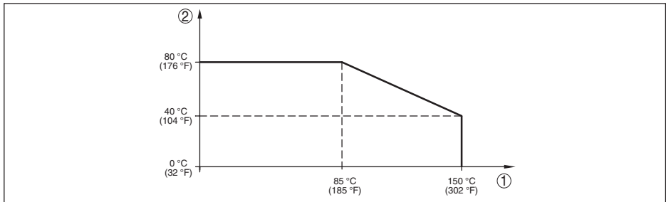
Fig. 26: Reducción de temperatura VEGABAR 83, versión hasta +150 °C (+302 °F)
