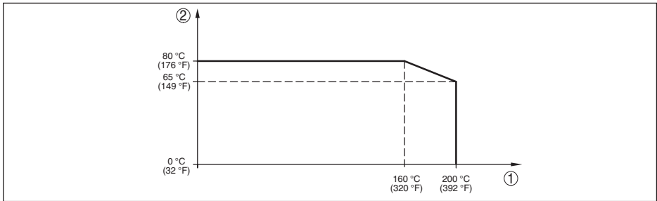
Fig. 29: Reducción de temperatura VEGABAR 83, versión hasta +200 °C (+392 °F)
