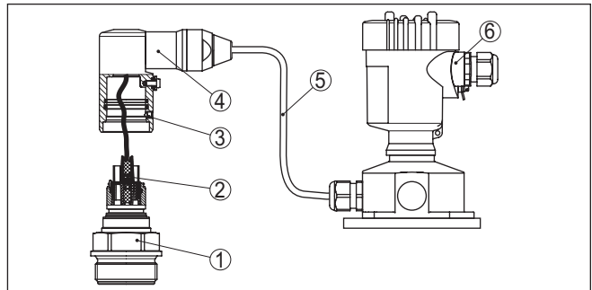
Fig. 21: VEGABAR 83 en versión IP68 25 bar y salida de cable lateral, carcasa externa
