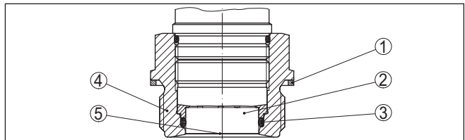
Fig. 4: Vlakke inbouw van de meetcel (voorbeeld: schroefdraad G1 \frac{1}{2} )
