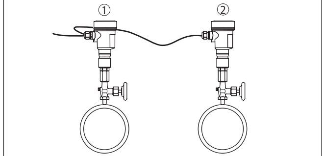
Fig. 15: Meetopstelling bij verschilddrukmeting van gasen in leidingen
