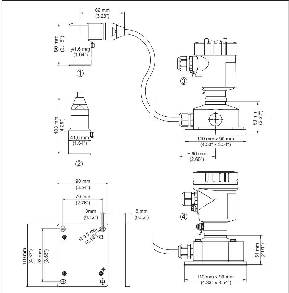
Fig. 37: VEGABAR 82, IP68-uitvoering met externe behuizing
