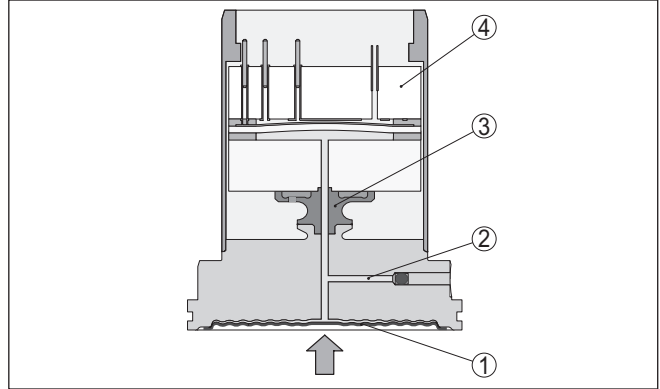
Fig. 3: Estructura de la celda de medición METEC® en VEGABAR 87
