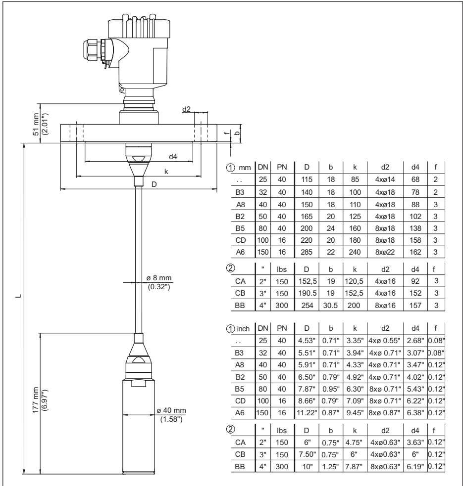
Fig. 41: VEGABAR 87, Conexión de brida
