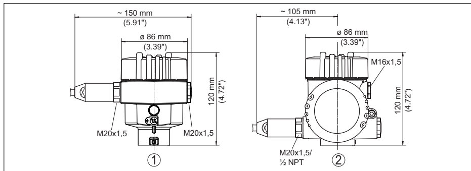
Fig. 35: Variantes de carcasa con tipo de protección IP66/IP68 (1 bar), (con el módulo de visualización y configuración montado aumenta la altura de la carcasa en 18 mm/0.71 in)
