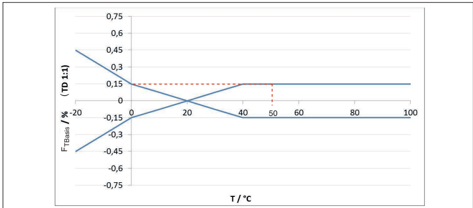
Fig. 32: Determinación del error de temperatura básica para el ejemplo anterior: F_{TBasis} = 0,15 \%
