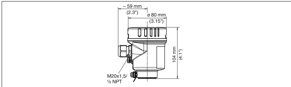
Fig. 38: Versión de carcasa en grado de protección IP69K (con módulo de visualización y configuración integrado aumenta la altura de la carcasa en 9 mm/0.35 in)
