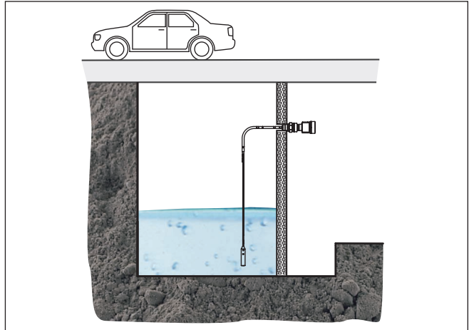
Abb. 18: Montage der Messsonde von der Seite
