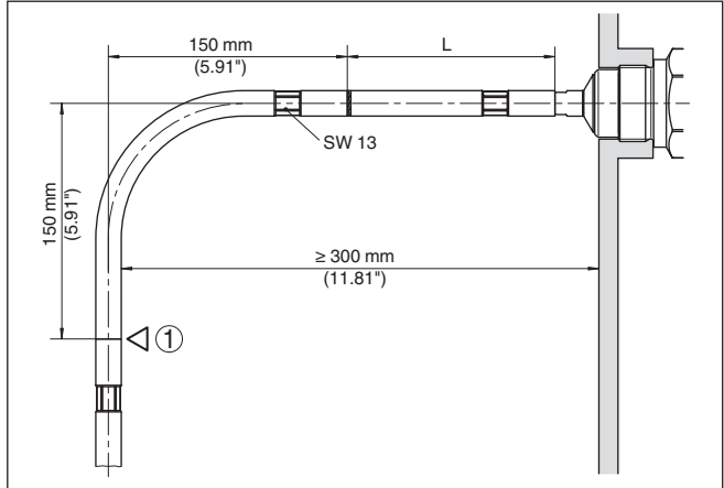
Abb. 4: Mindestabstand von der Behälterwand
