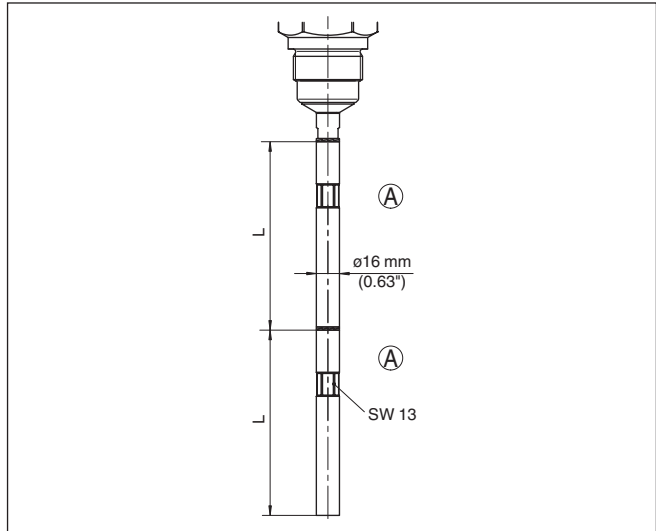
Abb. 23: Verlängerungsstäbe mit \varnothing 16 \text{ mm} (0.63 in)
