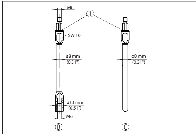
Abb. 8: Stabkomponenten mit \varnothing 8 \text{ mm} (0.315 in)
