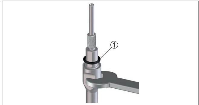
Abb. 7: Basisstab an den Prozessanschluss schrauben 1 Dichtungsring
