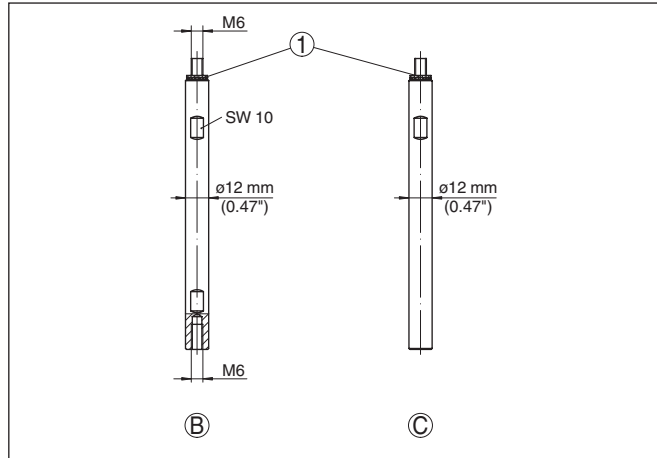
Abb. 14: Stabkomponenten mit \varnothing 12 mm (0.47 in)
