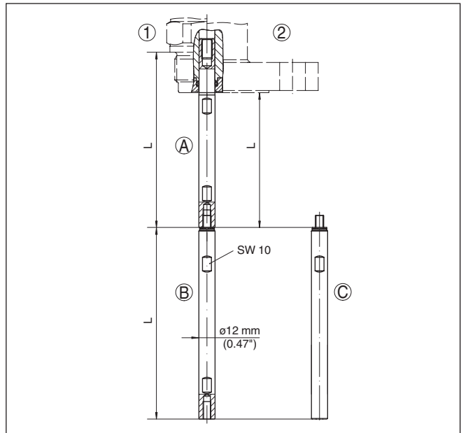
Abb. 9: Verlängerungsstäbe mit \varnothing 12 mm (0.47 in) - Bestelllänge der Messsonde
