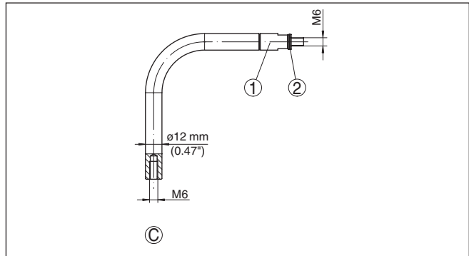
Abb. 13: Stabkomponenten mit \varnothing 12 mm (0.47 in) - Bogensegment
