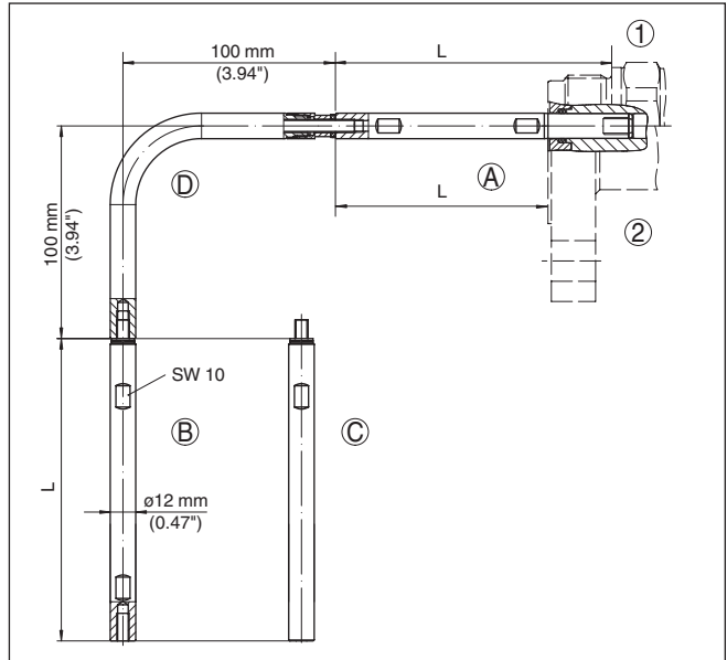
Abb. 10: Verlängerungsstäbe (Bogen) mit \varnothing 12 mm (0.47 in)
