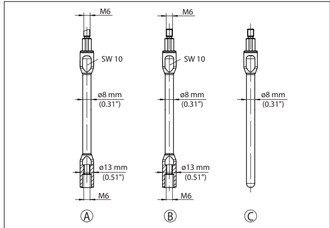
Abb. 1: Stabkomponenten mit \varnothing 8 \text{ mm} (0.315 in), poliert
