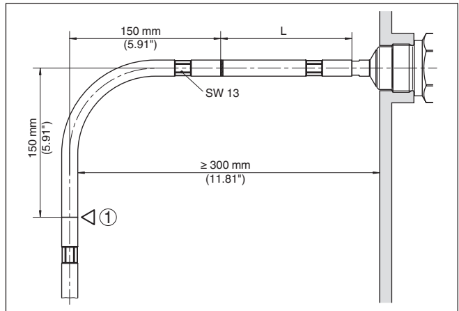
Abb. 5: Messbereich mit Bogensegment
