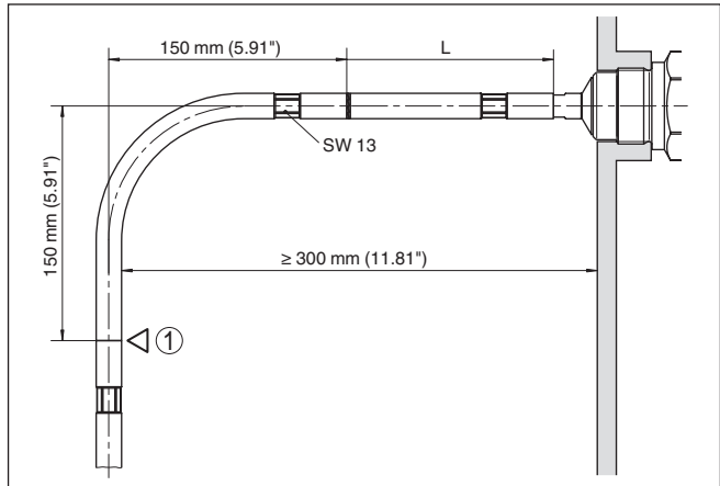
Abb. 24: Verlängerungsstäbe mit \varnothing 16 \text{ mm} (0.63 in)
