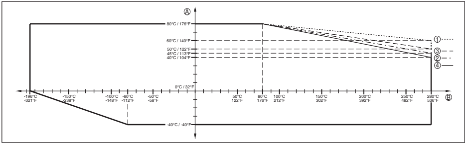
Abb. 37: Umgebungstemperatur - Prozesstemperatur, Standardausführung
