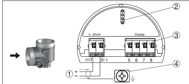
Abb. 12: Anschlussraum - Zweikammergehäuse
