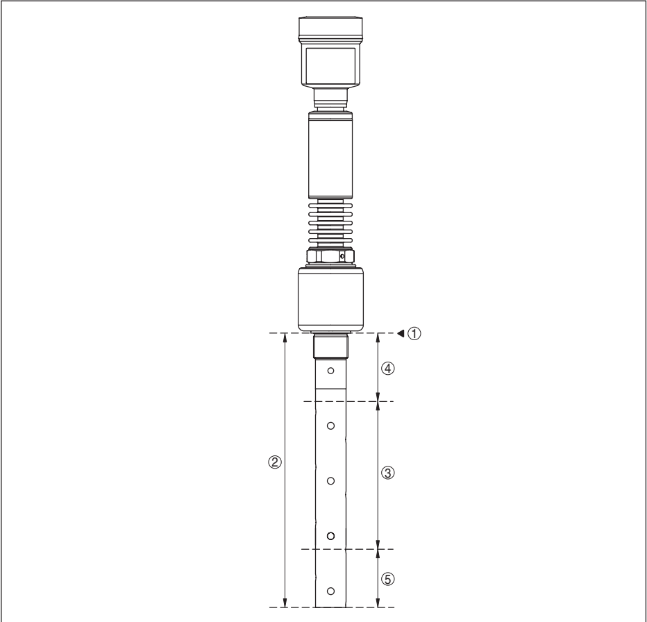
Abb. 31: Messbereiche - VEGAFLEX 86
