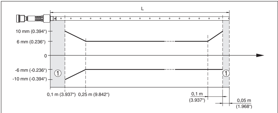
Abb. 35: Messabweichung VEGAFLEX 86 in Koaxialausführung in Medium Öl (Messlänge bis 6 m/19,69 ft)
