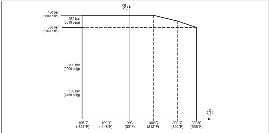
Abb. 39: Prozessdruck - Prozesstemperatur (Ausführung -196 ... +280 °C/-321 ... +536 °F)
