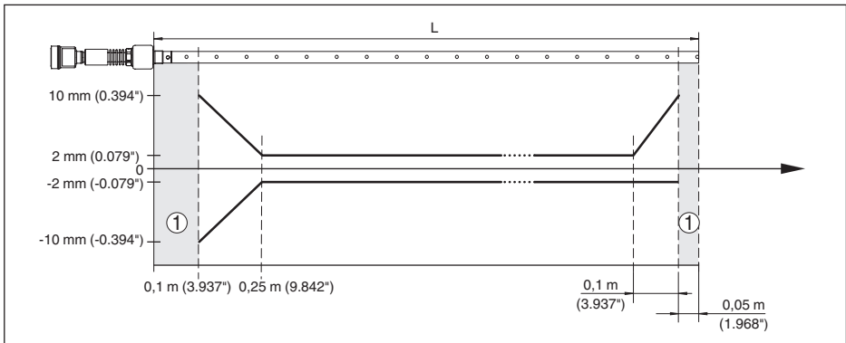
Abb. 34: Messabweichung VEGAFLEX 86 in Koaxialausführung in Medium Öl (Messlänge bis 1,5 m/4.92 ft)
