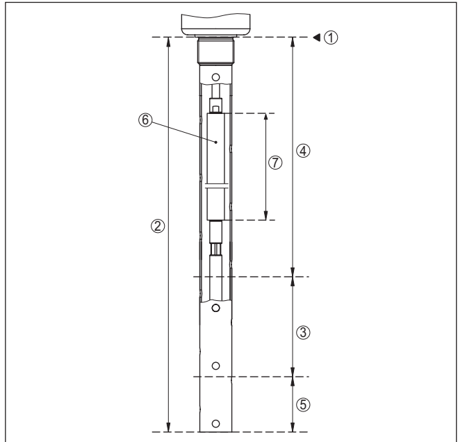
Abb. 8: Messbereiche - VEGAFLEX 86 mit Dampfkompensation
