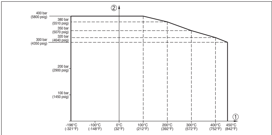
Abb. 40: Prozessdruck - Prozesstemperatur (Ausführung -196 ... +450 °C/-321 ... +842 °F)
