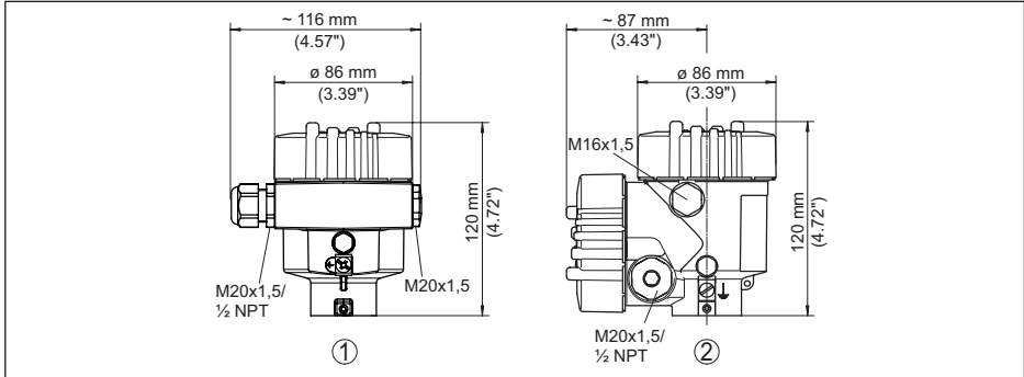
Abb. 42: Gehäuseausführungen in Schutzart IP66/IP68 (0,2 bar), (mit eingebautem Anzeige- und Bedienmodul vergrößert sich die Gehäusehöhe um 9 mm/0.35 in)
