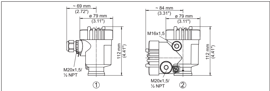
Abb. 41: Gehäuseausführungen in Schutzart IP66/IP67 (mit eingebautem Anzeige- und Bedienmodul vergrößert sich die Gehäusehöhe um 9 mm/0.35 in)
