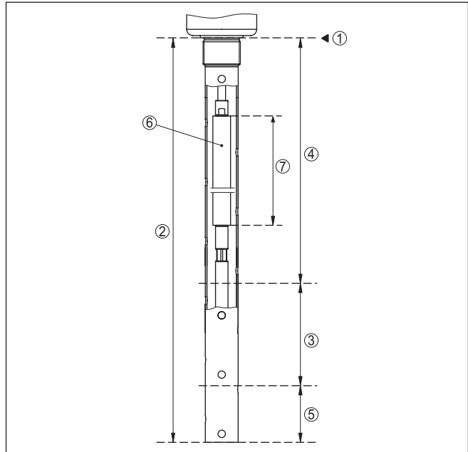
Abb. 36: Messbereiche - VEGAFLEX 86 mit Dampfkompensation
