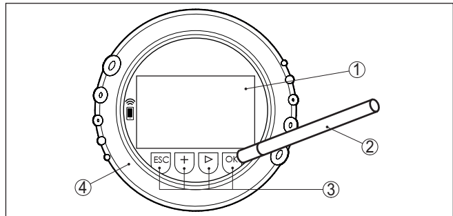
Abb. 22: Anzeige- und Bedienelemente - mit Bedienung über Magnetstift
