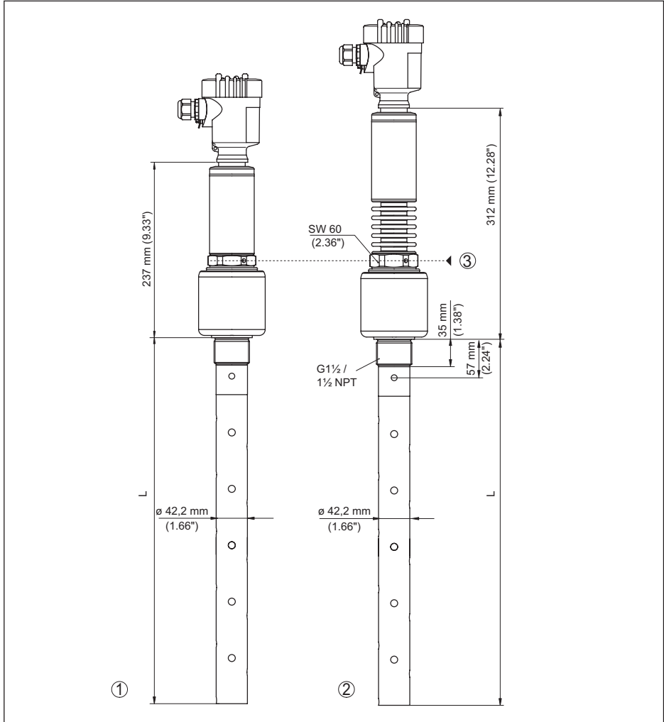
Abb. 46: VEGAFLEX 86, Gewindeausführung
