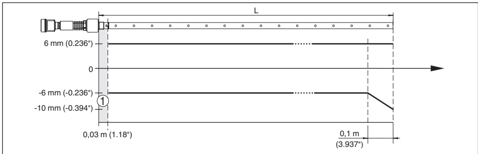
Abb. 33: Messabweichung VEGAFLEX 86 in Koaxialausführung in Medium Wasser (Messlänge bis 6 m/19.69 ft)
