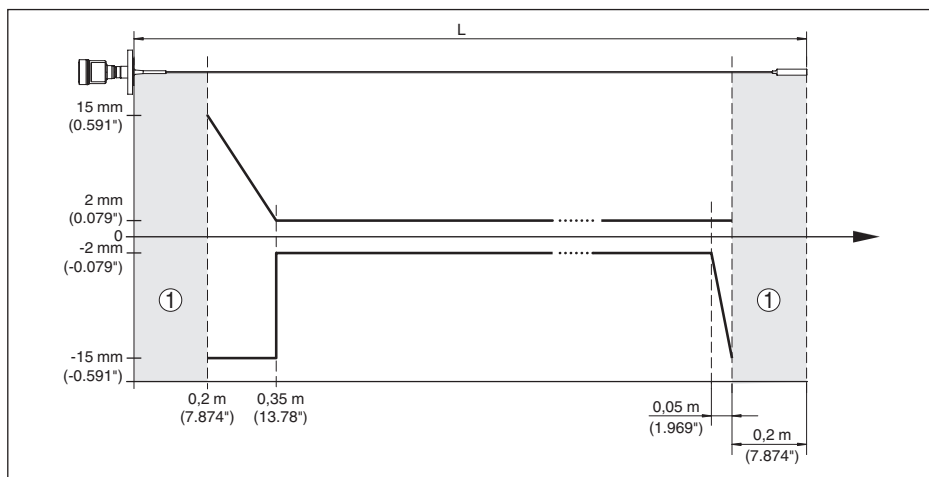
Rys. 33: Odchyłka pomiarowa VEGAFLEX 83 w wersji z falowodem linkowym (z powłoką) w przypadku napie- nienia zbiornika olejem
