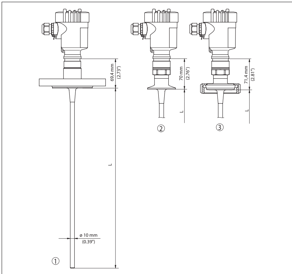
Rys. 41: VEGAFLEX 83, wersja z prętem
