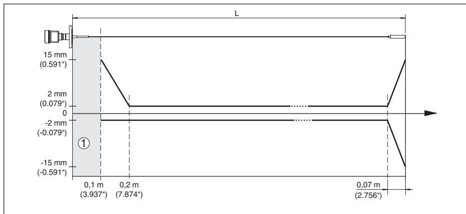
Rys. 32: Odchyłka pomiarowa VEGAFLEX 83 w wersji z falowodem linkowym (z powłoką) w przypadku napie- nienia zbiornika wodą
