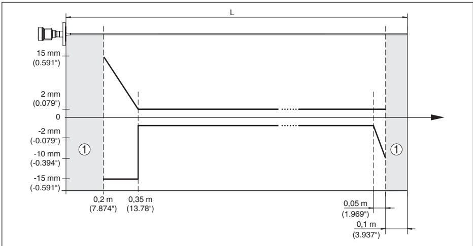
Rys. 31: Odchyłka pomiarowa VEGAFLEX 83 w wersji z falowodem prętowym (z powłoką) w przypadku napełnienia zbiornika olejem
