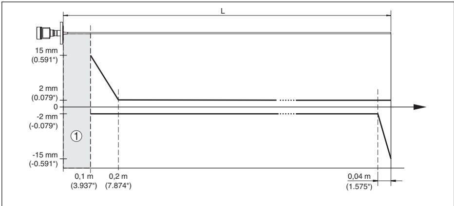
Rys. 30: Odchyłka pomiarowa VEGAFLEX 83 w wersji z falowodem prętowym (z powłoką) w przypadku napełnienia zbiornika wodą
