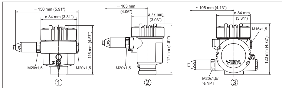
Rys. 39: Wersje wykonania obudowy ze stopniem ochrony IP66/IP68 (1 bar), (z zainstalowanym modułem wyświetlającym i obsługowym zwiększa się wysokość przyrządu o 9 mm/0.35 in)
