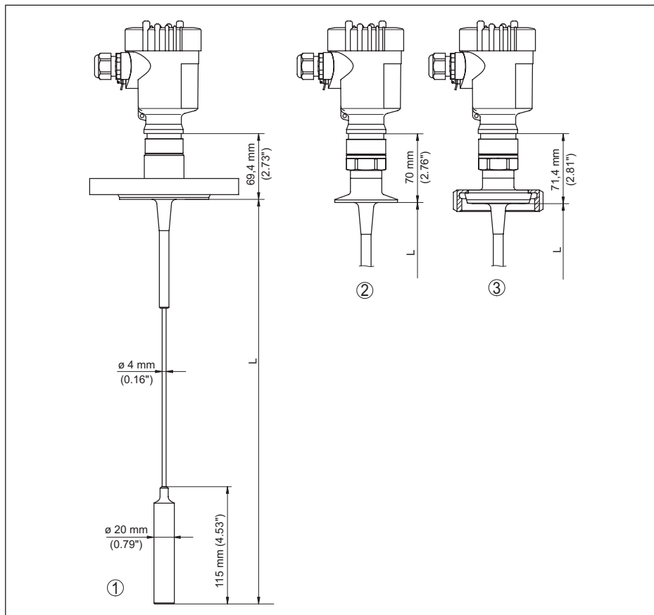
Rys. 40: VEGAFLEX 83, wersja z linką i obciążnikiem naprężającym
