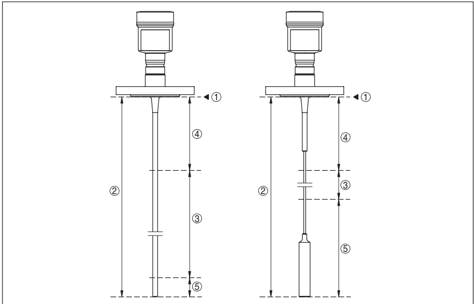
Figura 29: Campi di misura - VEGAFLEX 83
