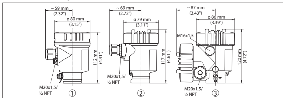
Figura 38: Le differenti custodie con grado di protezione IP66/IP68 (0,2 bar), (con tastierino di taratura con display incorporato l'altezza della custodia aumenta di 9 mm/0.35 in)
