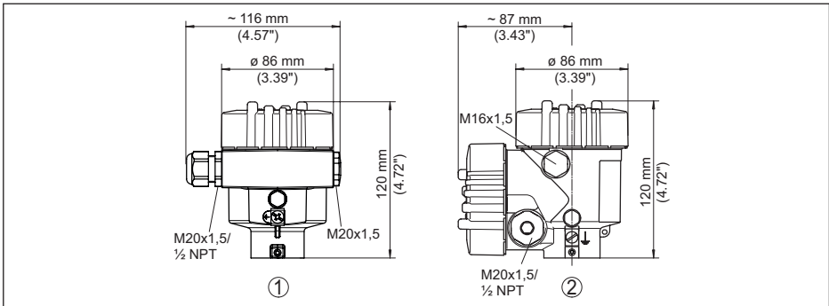
Figura 36: Le differenti custodie con grado di protezione IP66/IP68 (0,2 bar), (con tastierino di taratura con display incorporato l'altezza della custodia aumenta di 9 mm/0.35 in)
