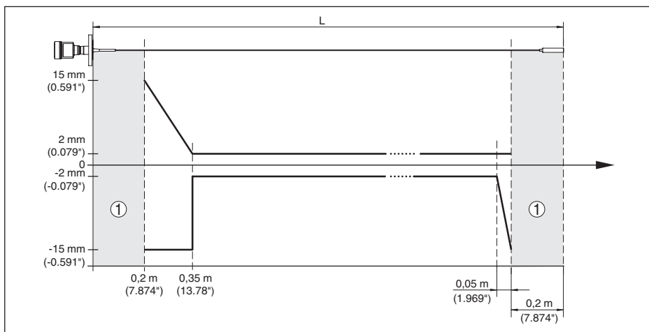
Figura 33: Scostamento di misura VEGAFLEX 83 in esecuzione a fune (rivestita) in olio
