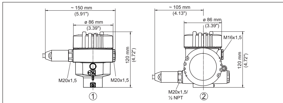
Figura 37: Le differenti custodie con grado di protezione IP66/IP68 (1 bar), (con tastierino di taratura con display incorporato l'altezza della custodia aumenta di 9 mm/0.35 in)
