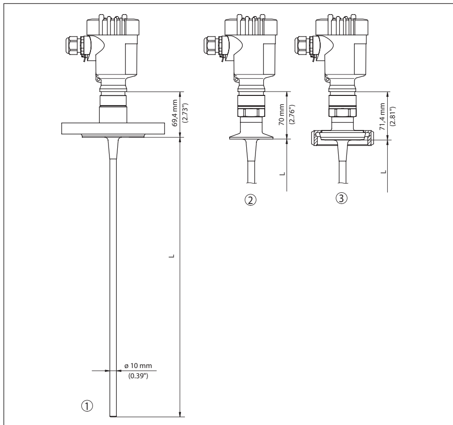
Figura 41: VEGAFLEX 83, esecuzione a barra
