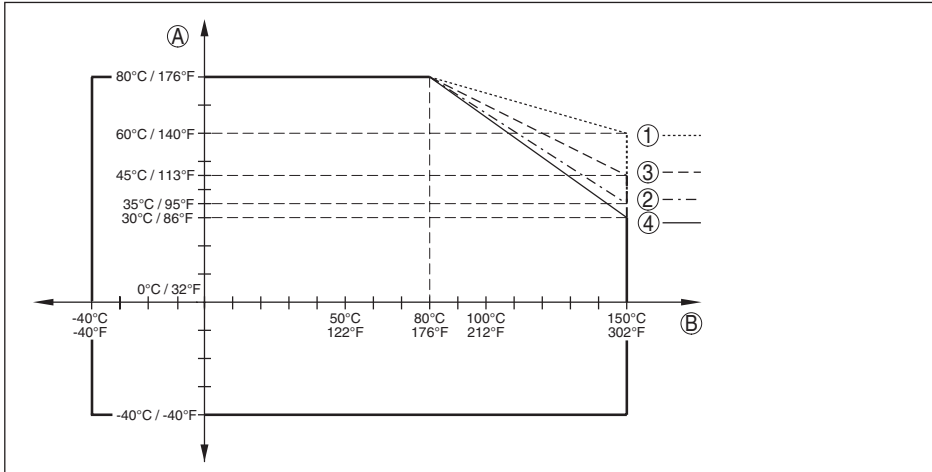
Figura 34: Temperatura ambiente - temperatura di processo, esecuzione standard
