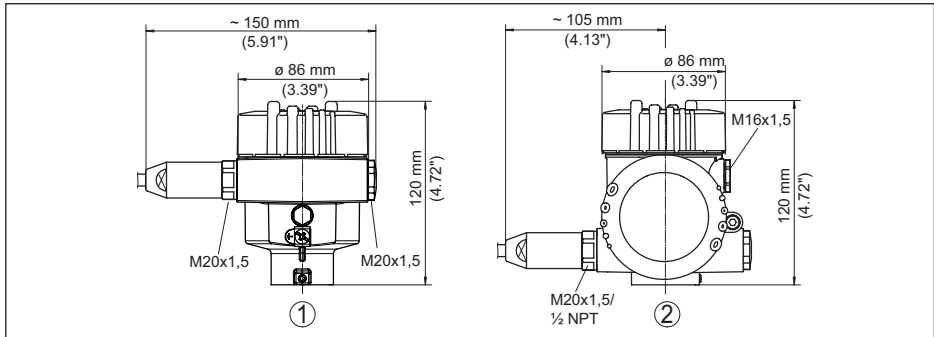
Fig. 35: Variantes de boîtier en protection IP66/IP68 (1 bar), (avec un module de réglage et d'affichage intégré, la hauteur du boîtier augmente de 9 mm/0.35 in)
