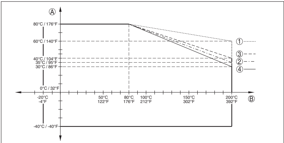
Fig. 32: Température ambiante - température process, version avec extension haute température
