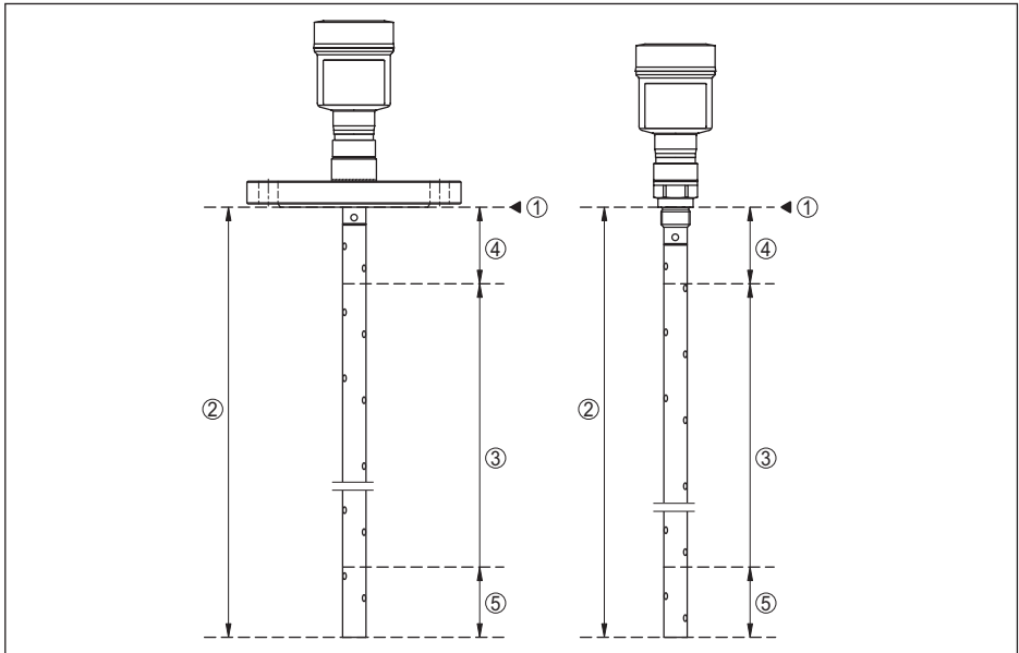
Fig. 28: Plages de mesure - VEGAFLEX 81
