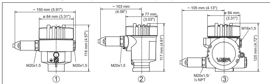
Fig. 37: Variantes de boîtier en protection IP66/IP68 (1 bar), (avec un module de réglage et d'affichage intégré, la hauteur du boîtier augmente de 9 mm/0.35 in)
