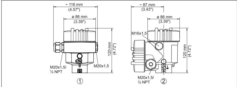
Fig. 34: Variantes de boîtier en protection IP66/IP68 (0,2 bar), (avec un module de réglage et d'affichage intégré, la hauteur du boîtier augmente de 9 mm/0.35 in)
