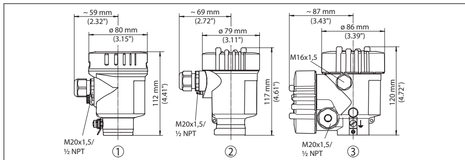
Fig. 36: Variantes de boîtier en protection IP66/IP68 (0,2 bar), (avec un module de réglage et d'affichage intégré, la hauteur du boîtier augmente de 9 mm/0.35 in)
