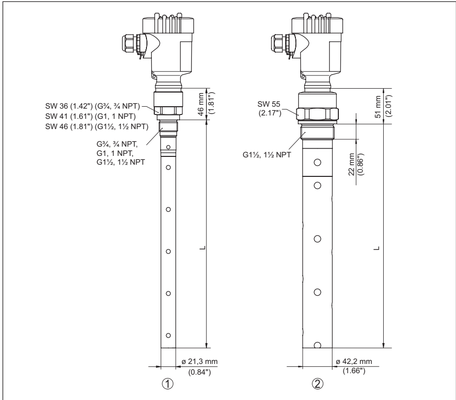
Abb. 38: VEGAFLEX 81, Gewindeausführung
