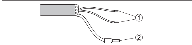
Abb. 14: Aderbelegung fest angeschlossenes Anschlusskabel
