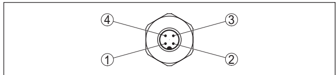
Abb. 13: Sicht auf den M12 x 1-Steckverbinder
