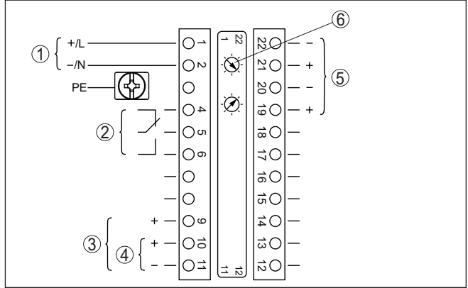
Res. 11: Ex olmayan cihazlar ve bünyesinde güvenliği olmayan akım çıkışlı cihazlarda elektronik bölme ve bağlantı bölmesi
