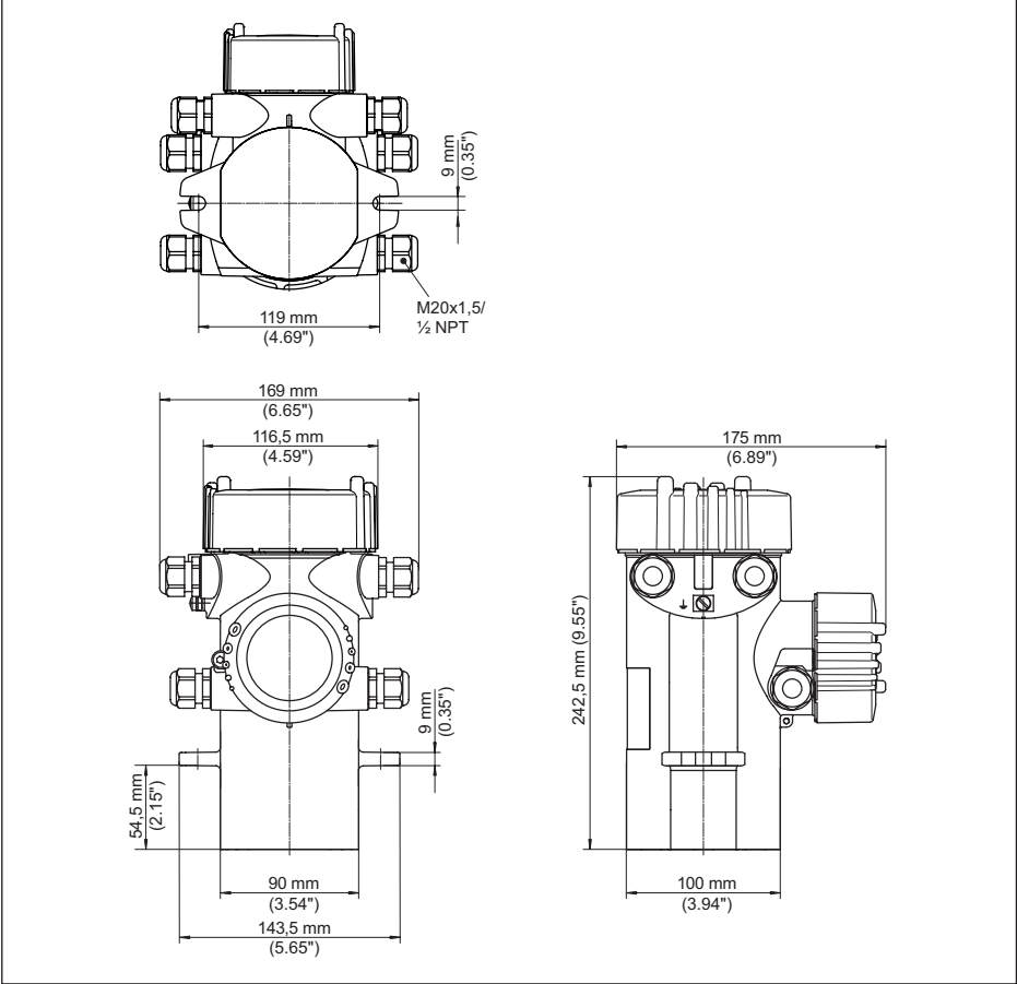
Res. 23: Alüminyum gövde ya da paslanmaz çelik gövde (hassas döküm)
