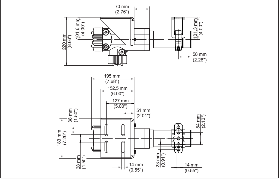
Res. 25: Dedektör borusu olan POINTRAC 31, 152 mm veya 304 mm (6 in/12 in) - montaj aksesuarı teslimat kapsamındadır
