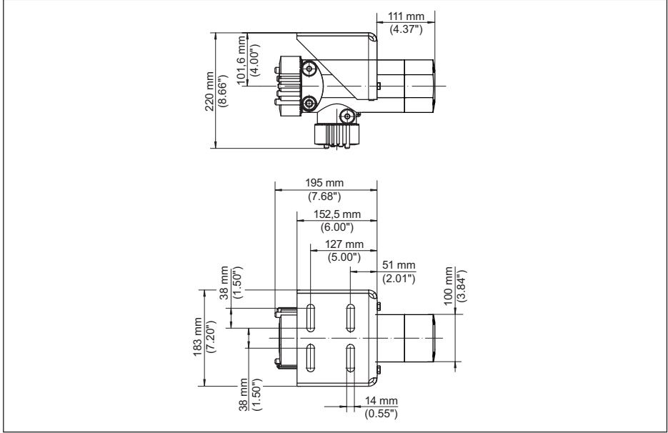
Res. 27: Dedektör borusu olmayan POINTRAC 31, 46 mm (1.8 in - montaj aksesuarı teslimat kapsamındadır
