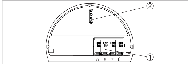
Res. 12: Ex olmayan cihazlar ve bünyesinde güvenliği olmayan akım çıkışlı cihazlarda kumanda ve bağlantı bölmesi
