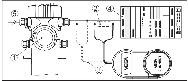
Res. 19: Bilgisayarı HART üzerinden sinyal hattına bağlanması
