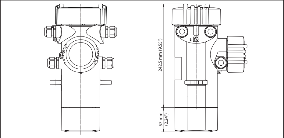
Res. 26: Dedektör borusu olmayan POINTRAC 31 - ölçüm aralığı = ısımarlanan uzunluk 46 mm (1.8 in)
