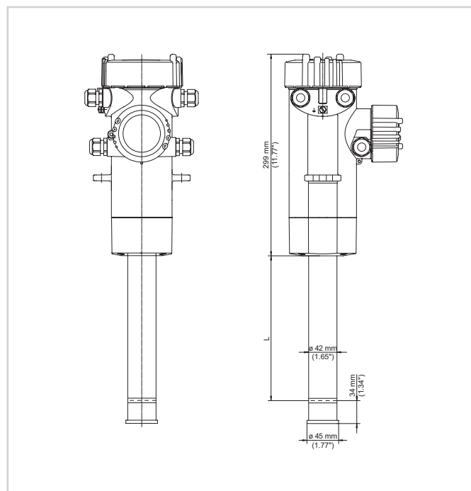
Dimensões FIBERTRAC 31
