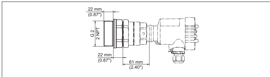
Fig. 37: Adaptador de montaje con tapa de cerámica (opcional) para VEGAMIP 62 con antena de trompeta interior, versión roscada G1½ con tapa de PTFE (también con rosca 1½ NPT)
