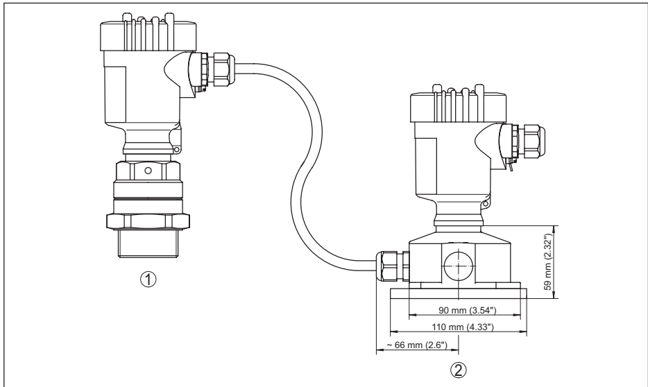
Fig. 33: Carcasa externa, unidad receptora
