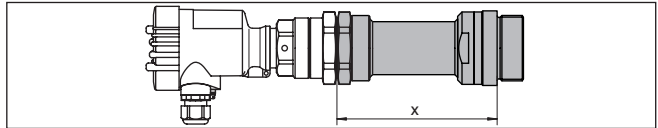
Fig. 14: VEGAMIP 62 con adaptador de montaje "Alta temperatura" -40 ... +450 °C (-40 ... +842 °F)
