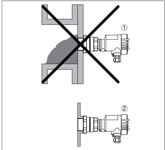
Fig. 11: Montaje rasante
