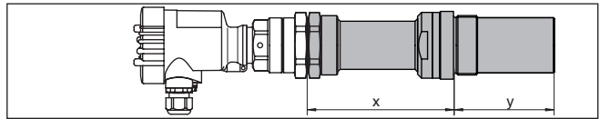
Fig. 5: VEGAMIP 62 con adaptador de montaje "Alta temperatura con tubo" -40 ... +450 °C (-40 ... +842 °F)
