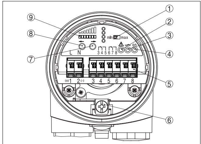
Fig. 27: Módulo electrónico MP6X R (unidad receptora) - Salida de relé
