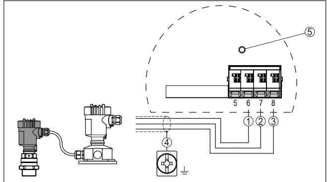
Fig. 24: Conexión de la línea hacia la carcasa externa (Unidad evaluadora)
