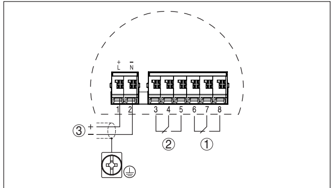
Fig. 26: Esquema de conexión unidad evaluadora - VEGAMIP 62 (Receiver)
