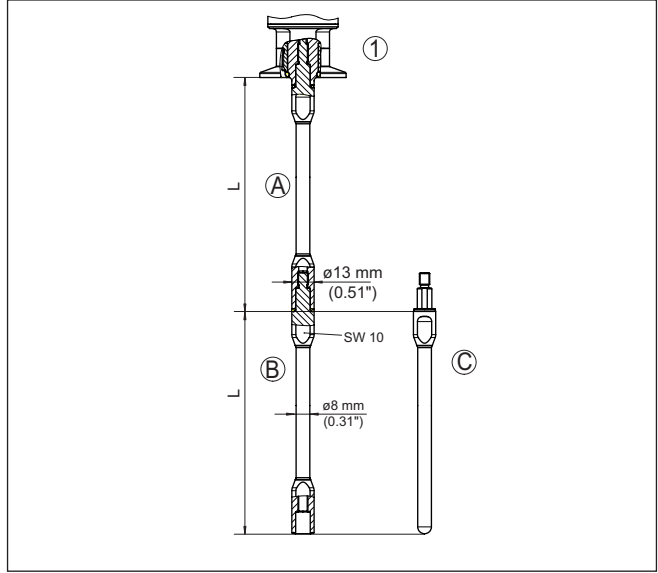
Res. 49: Uzatma çubukları - \varnothing 8 mm (0,315 in)
