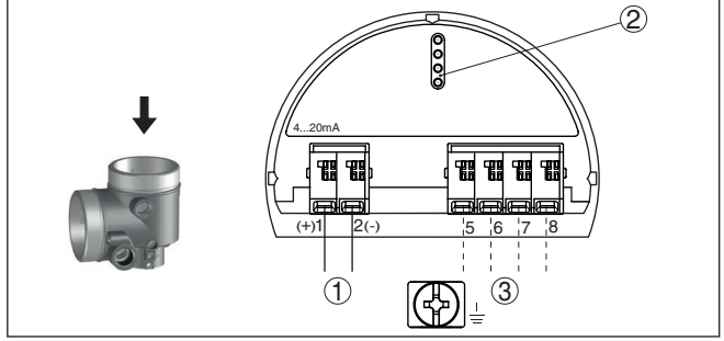
Res. 15: Elektronik bölümü - Ex d ia iki hücreli gövde
