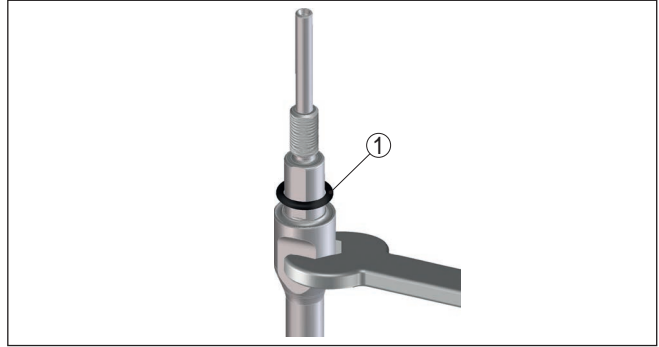
Res. 35: Ölçüm çubuğunu değiştir
