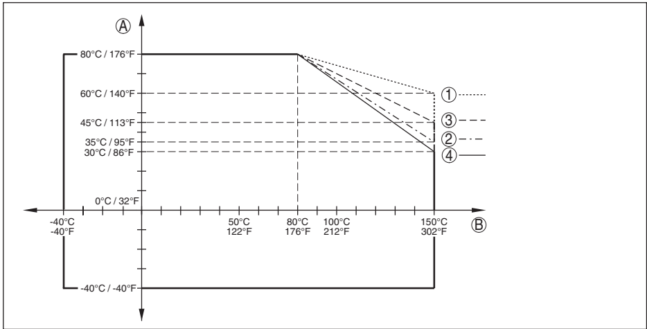
Res. 41: Ortam sıcaklığı - Proses sıcaklığı, standart model
