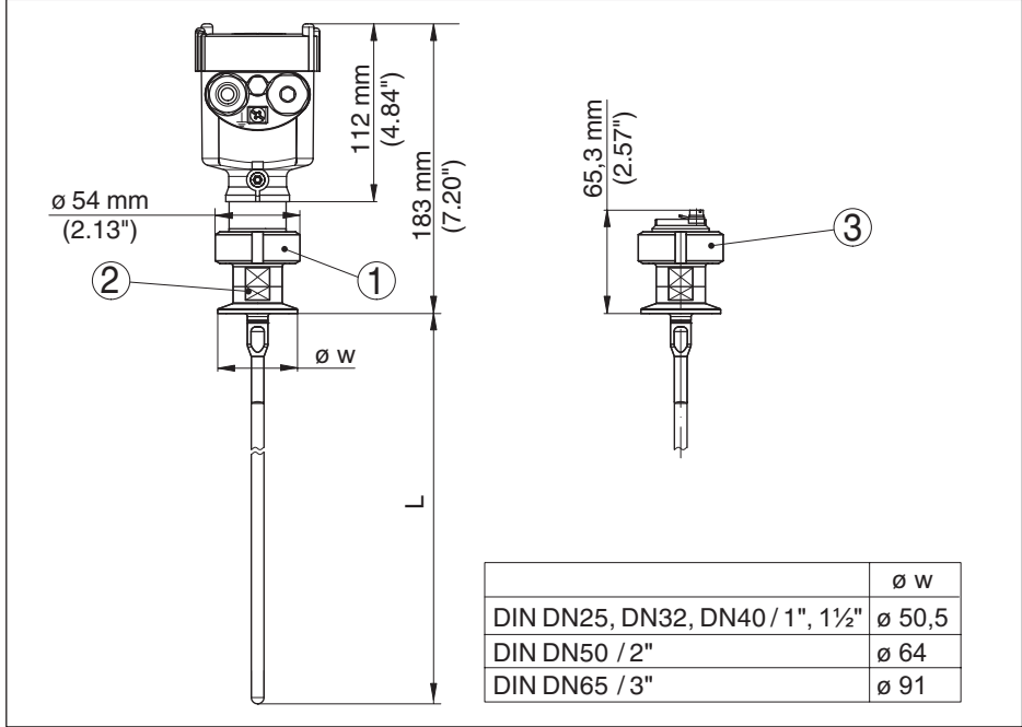
Res. 48: VEGAFLEX 83, çubuk model \varnothing 8 mm (0315 in), parlatılmış - Otoklavlanabilir model
