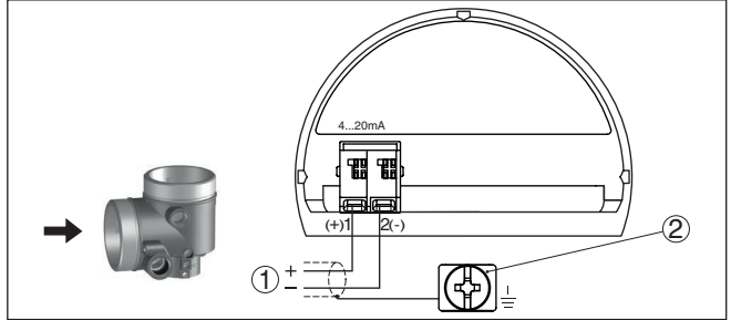
Res. 16: Ex d ia iki hücreli gövde - bağlantı bölümü
