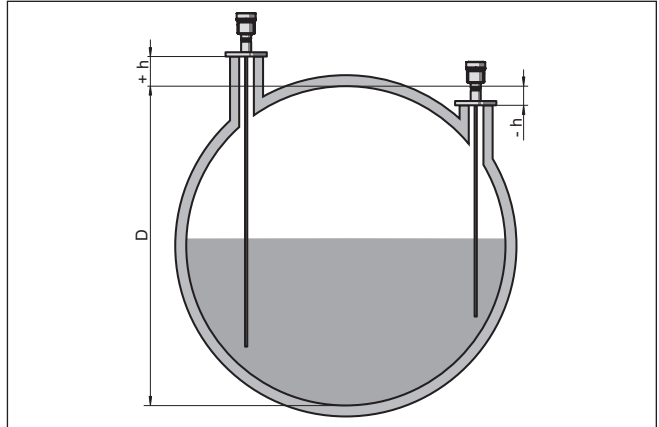
Rys. 25: Wysokość zbiornika i wartość korekcyjna położenia króćca
