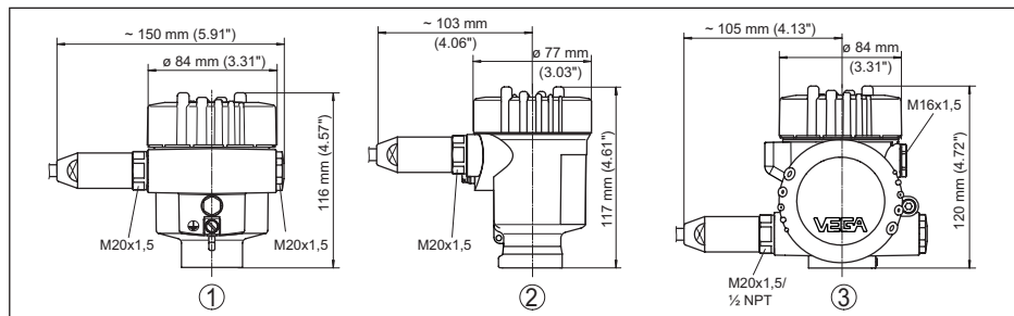
Rys. 44: Wersje wykonania obudowy ze stopniem ochrony IP66/IP68 (1 bar), (z zainstalowanym modułem wyświetlającym i obsługowym zwiększa się wysokość przyrządu o 9 mm/0.35 in)
