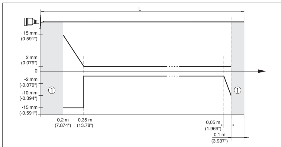
Rys. 36: Odchyłka pomiarowa VEGAFLEX 83 w wersji z falowodem prętowym (z powłoką) w przypadku napęnienia zbiornika olejem
