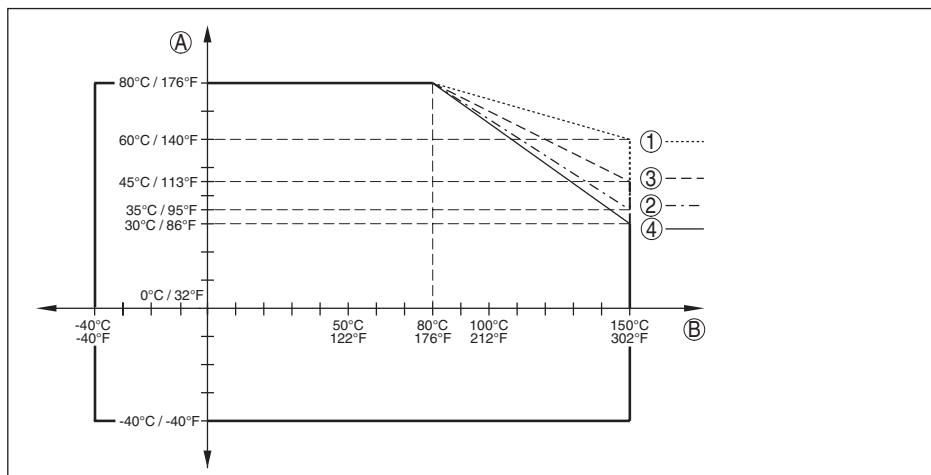
Rys. 39: Temperatura otoczenia - technologiczna, wersja standardowa
