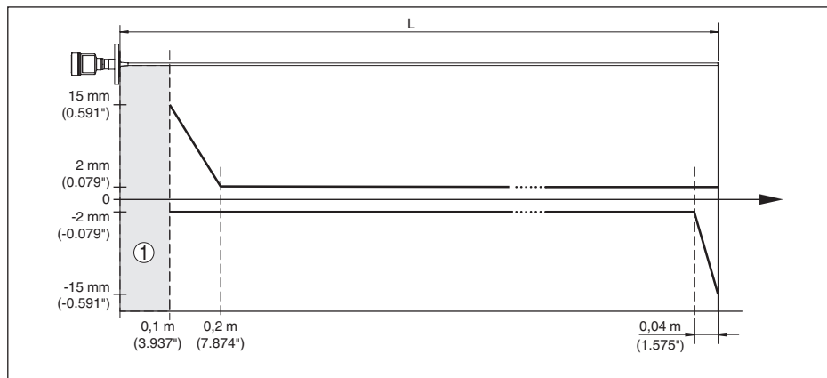
Rys. 35: Odchyłka pomiarowa VEGAFLEX 83 w wersji z falowodem prętowym (z powłoką) w przypadku napęnienia zbiornika wodą
