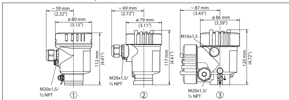
Rys. 43: Wersje wykonania obudowy ze stopniem ochrony IP66/IP68 (0,2 bar), (z zainstalowanym modułem wyświetlającym i obsługowym zwiększa się wysokość przyrządu o 9 mm/0.35 in)
