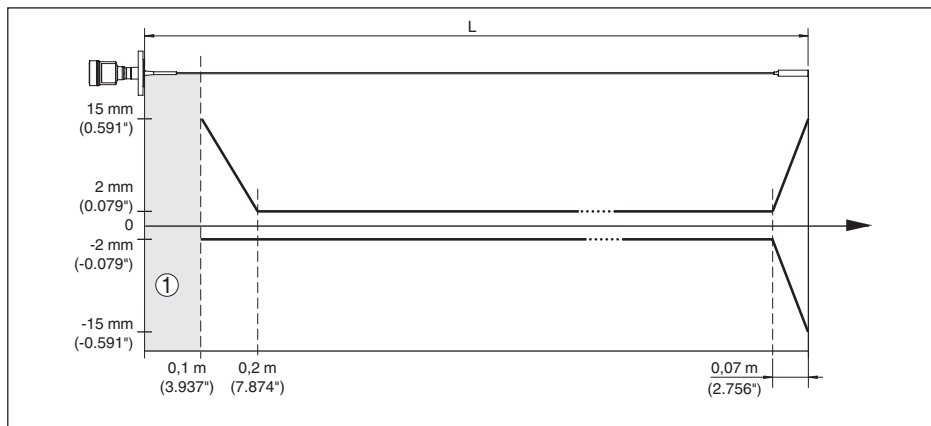
Rys. 37: Odchyłka pomiarowa VEGAFLEX 83 w wersji z falowodem linkowym (z powłoką) w przypadku napie- nienia zbiornika wodą
