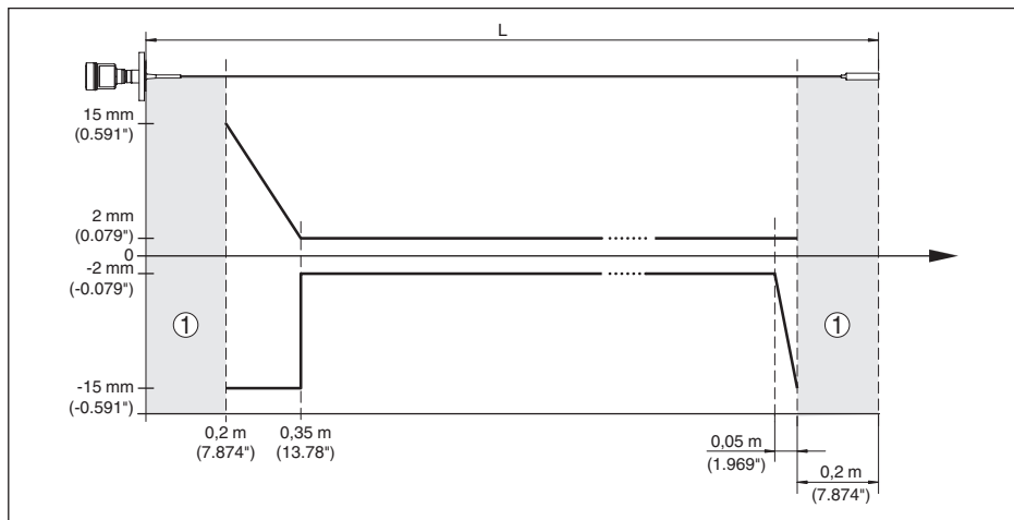
Rys. 38: Odchyłka pomiarowa VEGAFLEX 83 w wersji z falowodem linkowym (z powłoką) w przypadku napie- nienia zbiornika olejem
