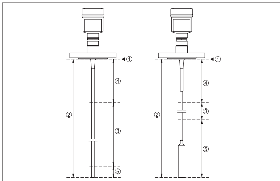
Rys. 34: Zakresy pomiarowe - VEGAFLEX 83
