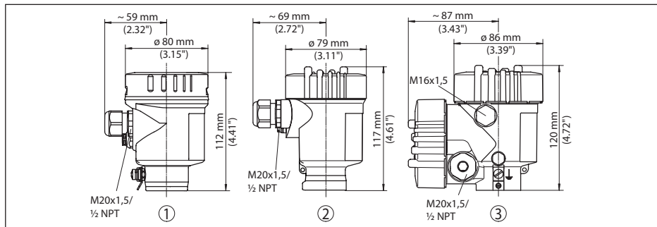
Fig. 43: Variantes de boîtier en protection IP66/IP68 (0,2 bar), (avec un module de réglage et d'affichage intégré, la hauteur du boîtier augmente de 9 mm/0.35 in)
