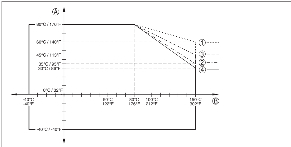
Fig. 39: Température ambiante - température process, version standard
