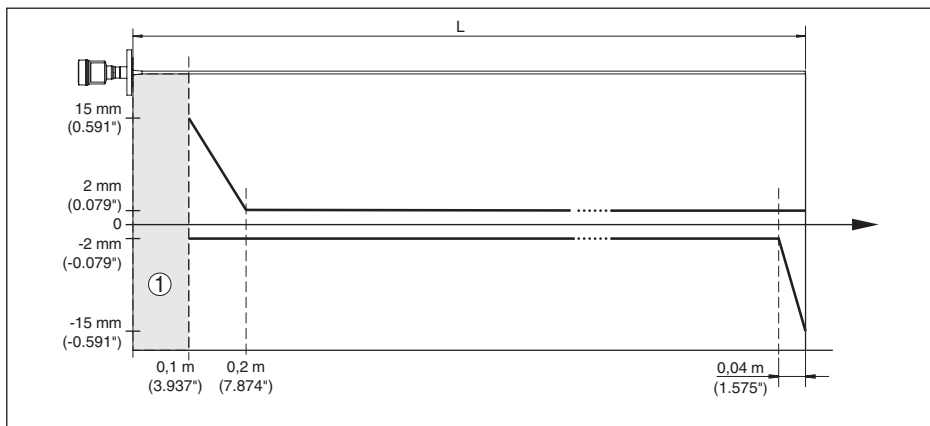
Fig. 35: Écart de mesure VEGAFLEX 83 en version tige (revêtue) dans l'eau
