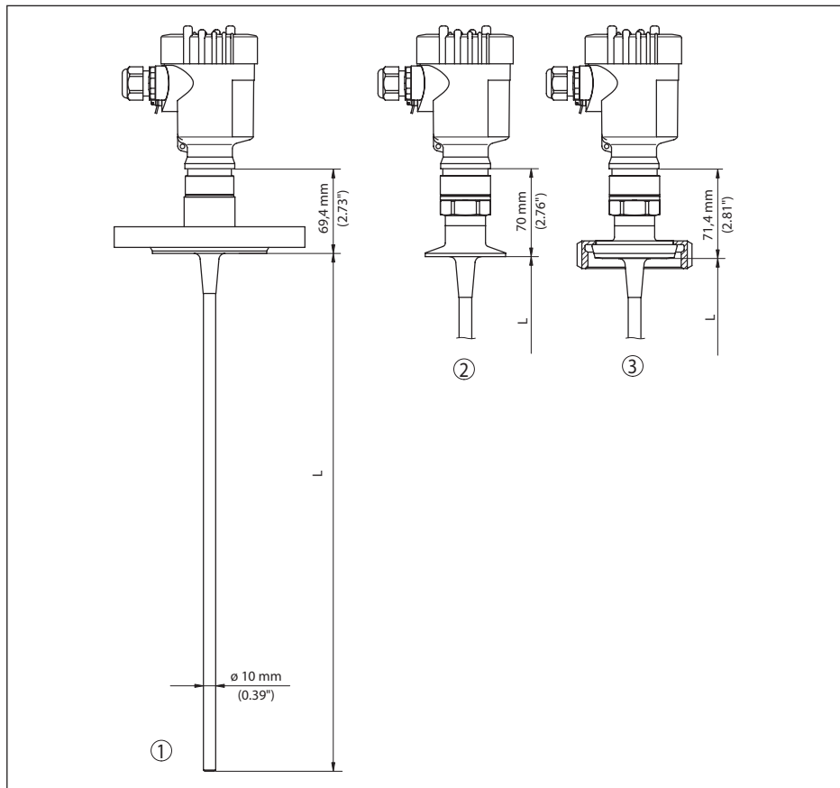
Fig. 46: VEGAFLEX 83, version tige
