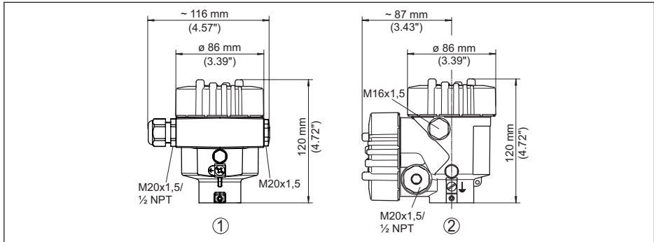
Fig. 41: Variantes de boîtier en protection IP66/IP68 (0,2 bar), (avec un module de réglage et d'affichage intégré, la hauteur du boîtier augmente de 9 mm/0.35 in)
