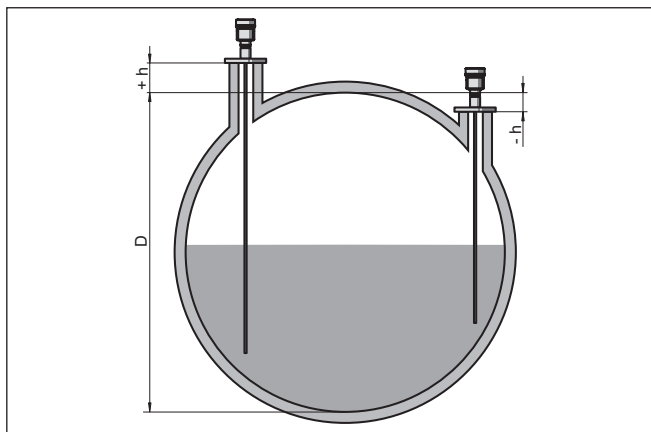
Fig. 25: Hauteur de la cuve et valeur de correction du manchon
