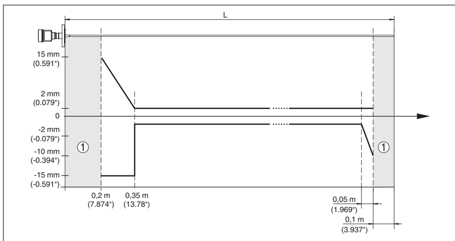
Fig. 36: Écart de mesure VEGAFLEX 83 en version tige (revêtue) dans l'huile
