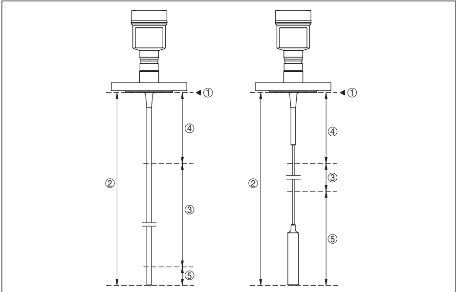
Fig. 34: Plages de mesure - VEGAFLEX 83
