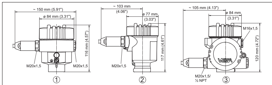
Fig. 44: Variantes de boîtier en protection IP66/IP68 (1 bar), (avec un module de réglage et d'affichage intégré, la hauteur du boîtier augmente de 9 mm/0.35 in)
