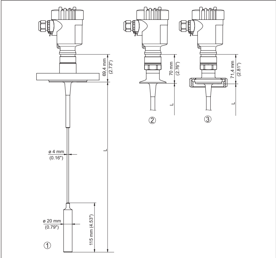
Fig. 45: VEGAFLEX 83, version câble avec poids tenseur
